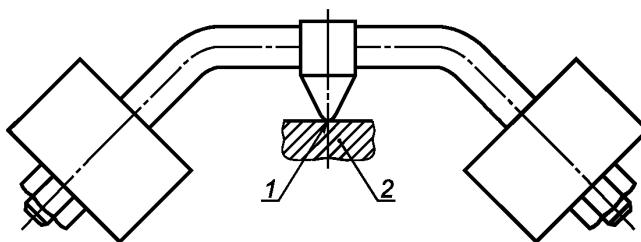
1 — сфера R = 2,5 \text{ мм} ; 2 — образец
