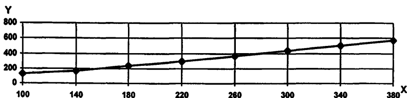
Рисунок Д.1-Зависимость нового числа твердости Hd, кгс/мм 2 (ось Y) от числа твердости по Бринеллю HB, кгс/мм 2 (ось X)
