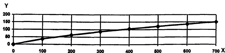
Рисунок Д.2 – Зависимость предела прочности, \sigma_B , кгс/мм 2 (ось Y) от нового числа твердости Hd, кгс/мм 2 (ось X)
