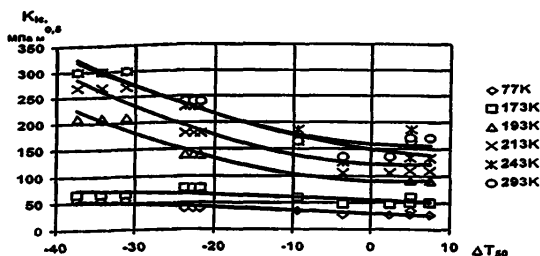
Рисунок 2 - Обобщенная зависимость между \Delta T_{50} и K_{Ic} для низколегированных и низкопрочных сталей
