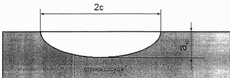
Рисунок 1- Параметры формализованного дефекта
