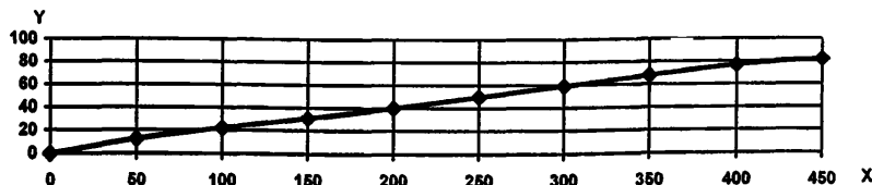
Рисунок Д.3 - Зависимость предела текучести, \sigma_{0,2} , кгс/мм 2 (ось Y) от нового числа твердости Hd, кгс/мм 2 (ось X)
