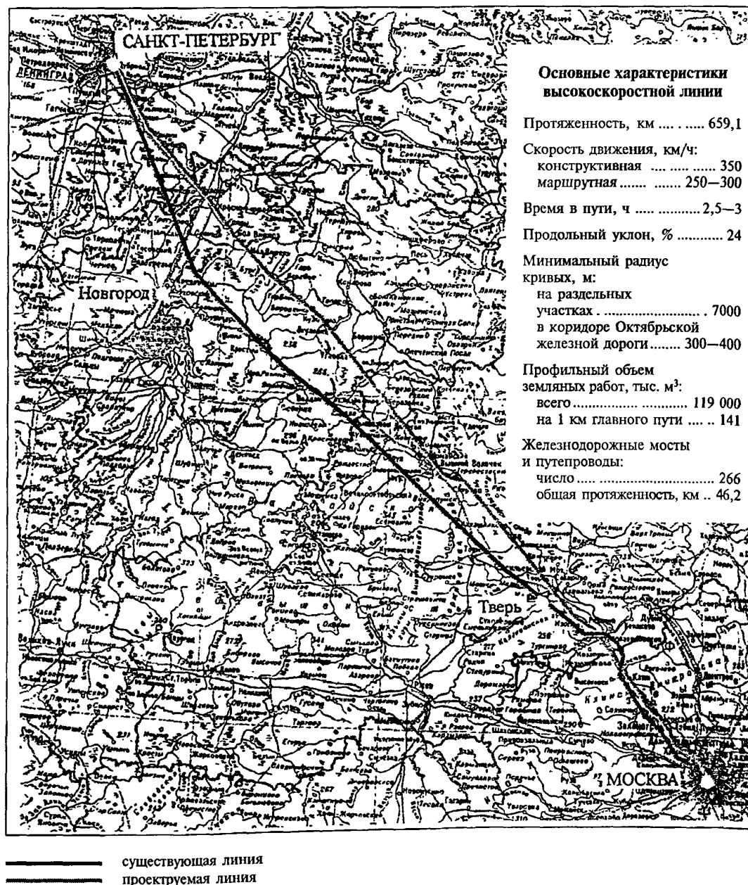
Рисунок 17 — Трассы высокоскоростной и существующей линий Москва—С.-Петербург (проект РАО «Высокоскоростные магистрали»)
