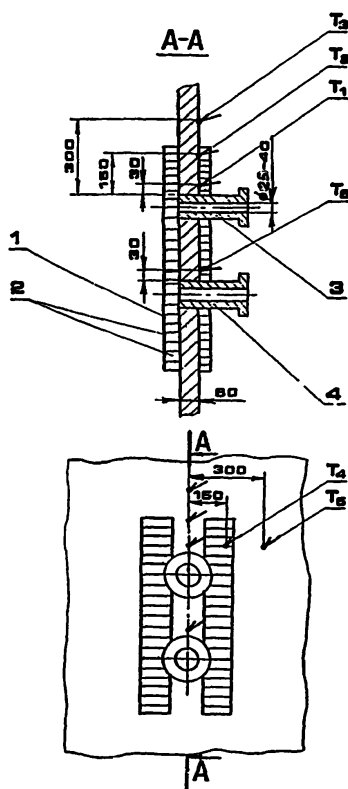
1-стенка корпуса ; 2-нагреватели; 3-термообрабатываемый штуцер; 4-соседний штуцер; T1-T6-термопреобразователи.
