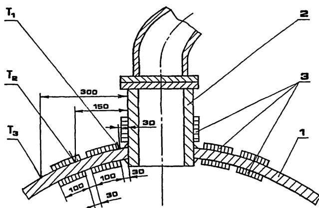
1 - верхнее днище; 2 - штуцер; 3 - нагреватели; T1 - T3 термопреобразователи
