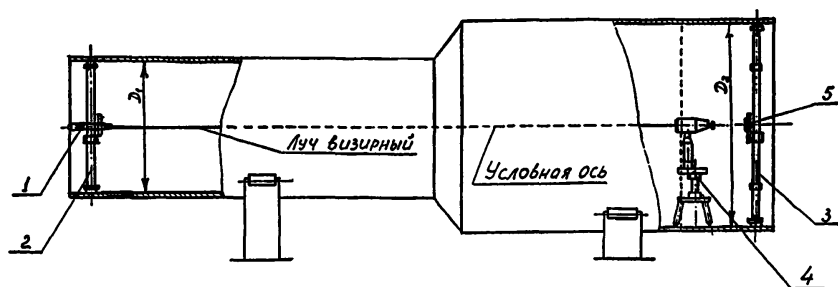
1- лазерный визир; 2-центратор D1; 3 – центратор D2;4- устройство для поворота луча на угол 90^\circ ; 5- мишень.
