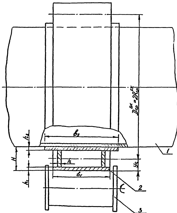
Рисунок Б.2 - Схема установки корпуса аппарата с бандажным кольцом на ролике роликоопоры
