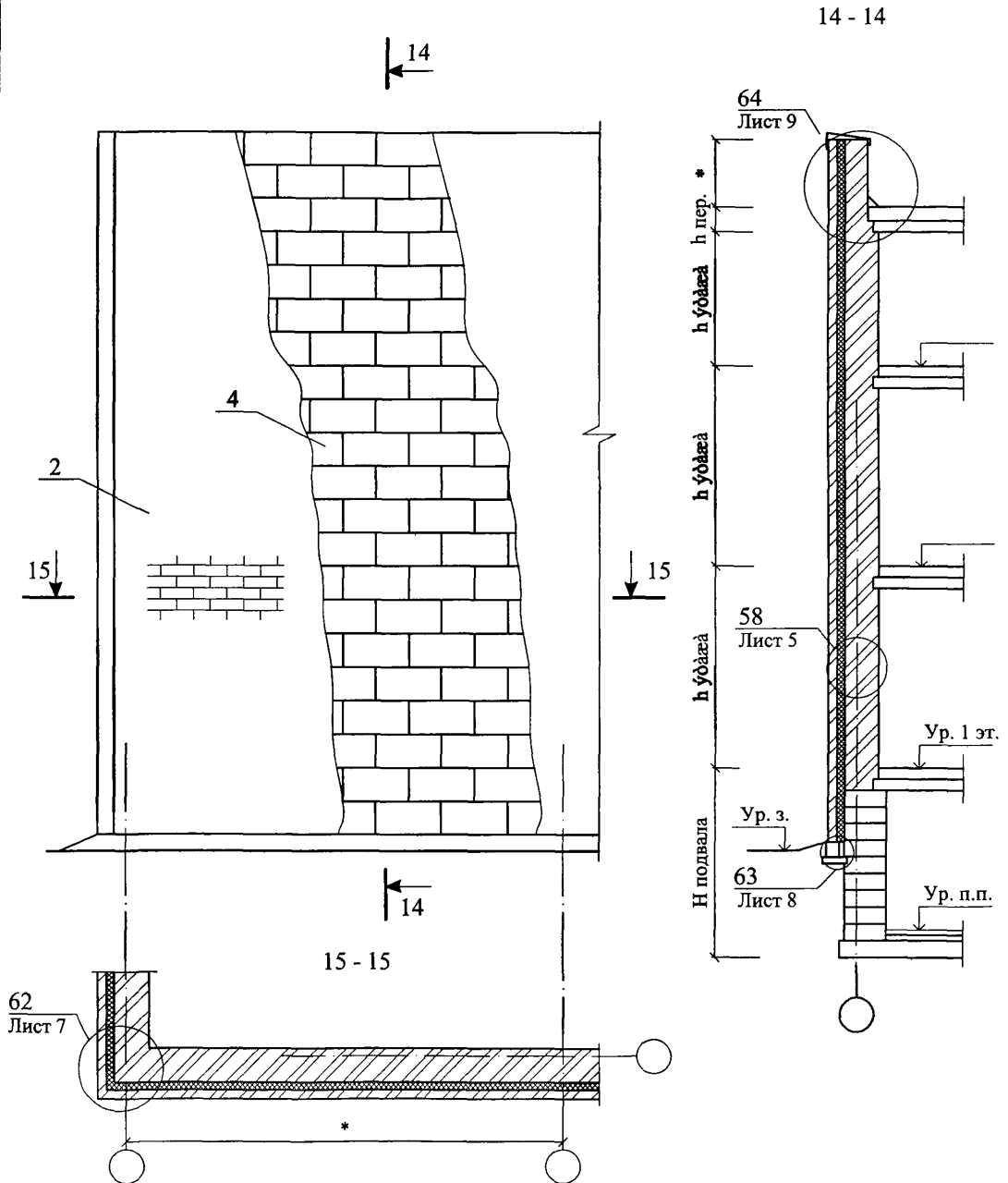
СХЕМА № 11. Расположение плит утеплителя, рассечек
