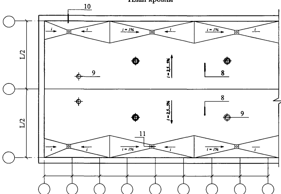
План кровли
