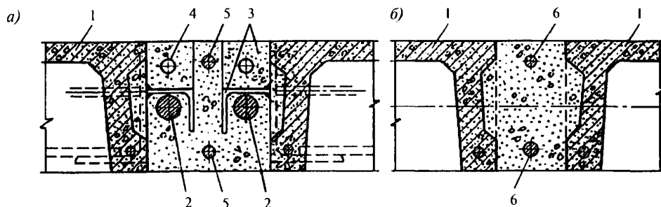
а — узел опирания железобетонных плит на контурные ванты; б — поперечное сечение продольного ребра оболочки (балки); 1 — железобетонные ребристые плиты; 2 — контурные ванты; 3 — крюк жесткой конструкции; 4 — отверстие для строповки плит; 5 — дополнительная арматура в поперечных швах оболочки; 6 — рабочая арматура продольных ребер (балок)
