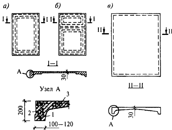
а — ступенчато-вспарушенная панель с одним кессоном; б — ступенчато-вспарушенная панель с двумя кессонами; в — вспарушенная панель; 1 — основная растянутая арматура пояса; 2 — каркас поперечного армирования контурного ребра; 3 — сетка плиты
