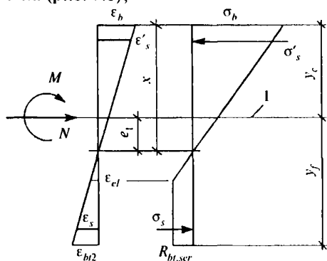
Рисунок 9.8 — Схема напряженно-деформированного состояния сечения оболочки при проверке образования трещин при действии изгибающего момента и нормальной силы
