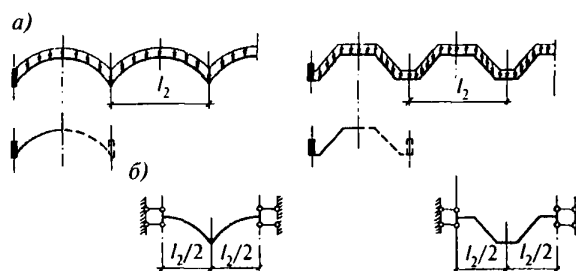
Рисунок 9.5 — К приближенному расчету многоволновых оболочек и складок
