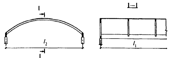
Рисунок 9.10 — Ребристая оболочка
