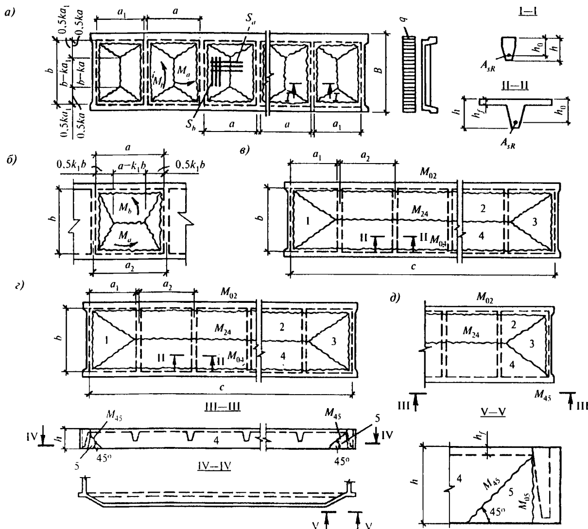
Рисунок 9.20 — Схемы разрушения полки и поперечных ребер плит от изгиба и продольных ребер от кручения
