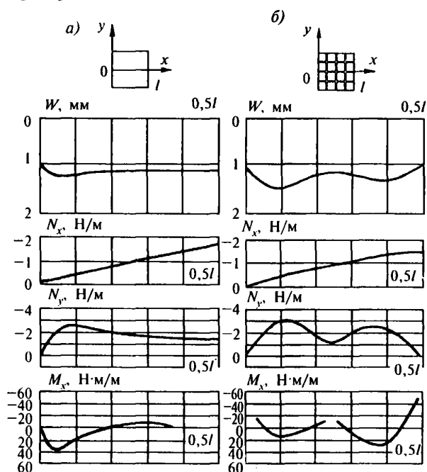
Рисунок 11.12 — Графики прогибов W и усилий N_x , N_y , M_x по результатам экспериментальных исследований моделей оболочек
