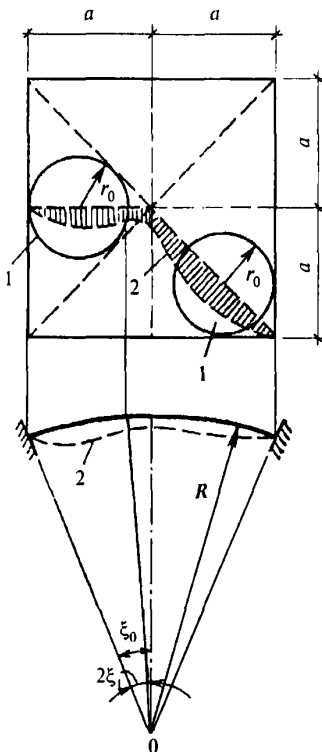
Рисунок 11.14 — Схема разрушения оболочки с образованием локальной вмятины
