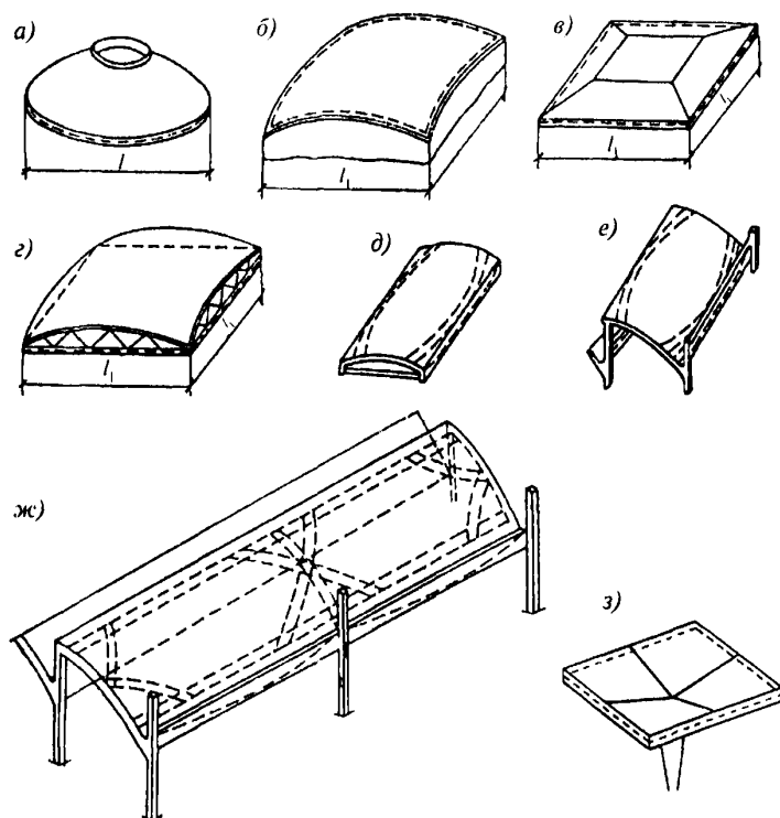
Рисунок 6.1 — Схемы расположения напрягаемой арматуры
