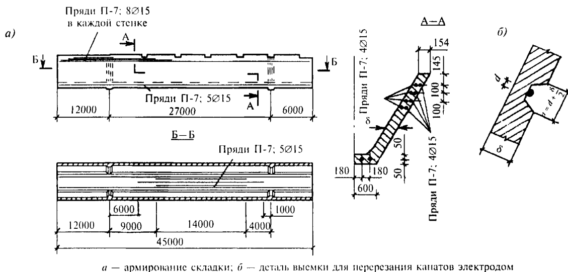
Рисунок 8.3 — Пример армирования консольно-балочной складки покрытия прямолинейной предварительно напряженной арматурой с обрывом канатов в соответствии с эпюрой моментов
