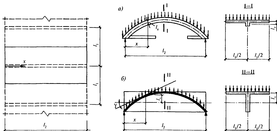
Рисунок 9.18 — К расчету диафрагмы короткой оболочки
