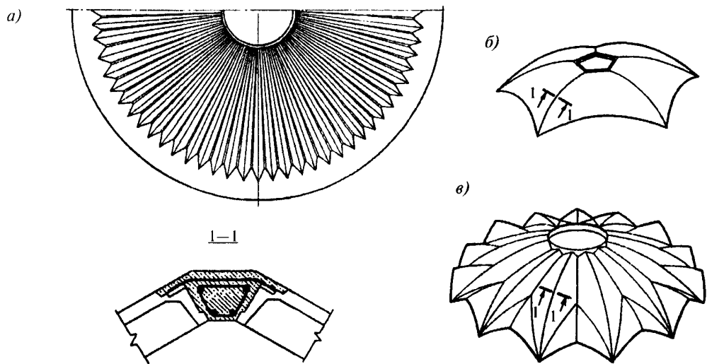
a — складчатый купол; б, в — сопряженные купольные оболочки Рисунок 10.10 — Формы купольных оболочек
