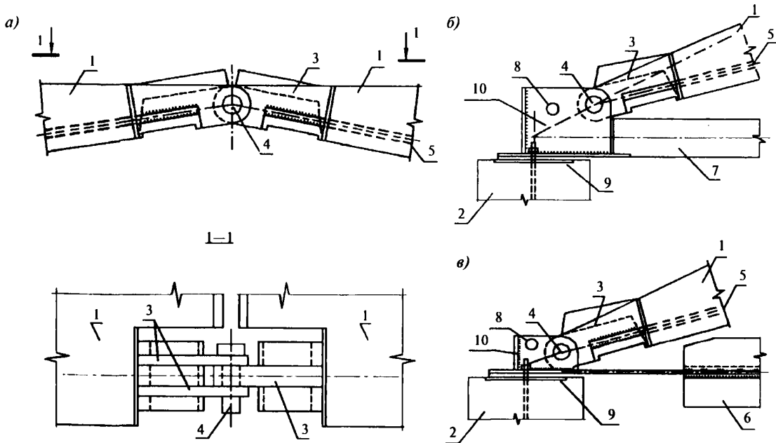
а — ключевой узел; б — опорный узел с железобетонными предварительно напряженными затяжками; в — опорный узел с затяжками из стального проката; 1 — панель-оболочка КЖС; 2 — опорная конструкция; 3 — закладные детали с отверстием для шарнира; 4 — металлический шарнир; 5 — арматура диафрагм плиты; 6 — затяжки из стального проката; 7 — преднапряженные железобетонные затяжки; 8 — отверстие для строповки свода; 9 — закладная деталь опорной конструкции; 10 — металлический упор затяжки
