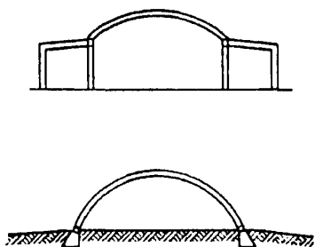
Рисунок 7.2 — Свод без затяжек
