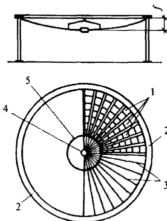
1 — плиты; 2 — опорный контур; 3 — ванты; 4 — центральное кольцо; 5 — опорное кольцо фонаря
