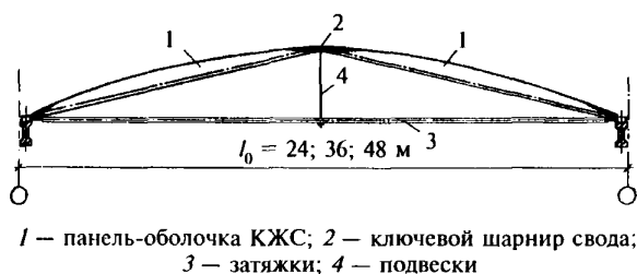
Рисунок 14.11 — Конструктивная схема сегментного свода для покрытий, опирающегося на продольные балки каркаса здания
