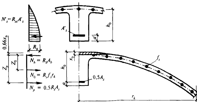
Рисунок 11.19 — Схема разрушения ребристой оболочки в зоне приложения сосредоточенной нагрузки
