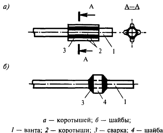
Рисунок 13.9 — Нерегулируемые анкеры вант из стержневой стали, выполняемые с помощью приваренных элементов
