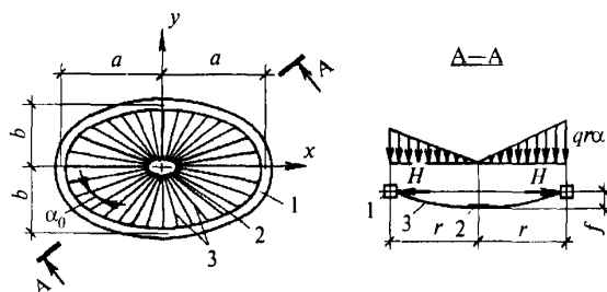
Рисунок 13.11 — Радиальная вантовая сеть с горизонтальной касательной в узле
