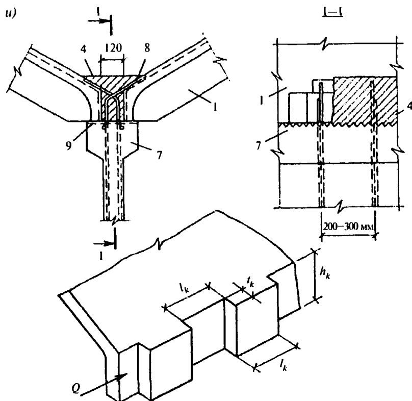
Рисунок 6.5 — Схема стыков сборных конструкций
