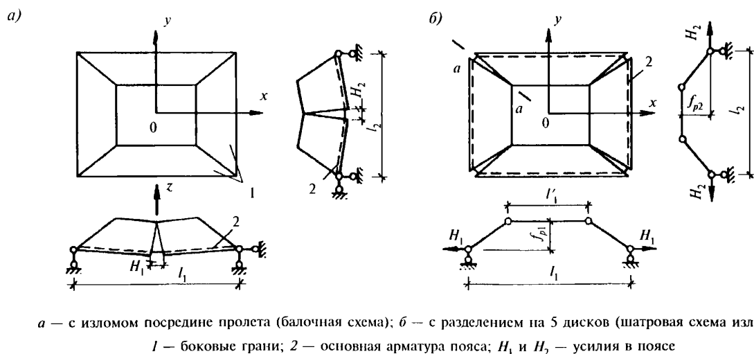
Рисунок 16.3 — Схемы разрушения шатровых складок
