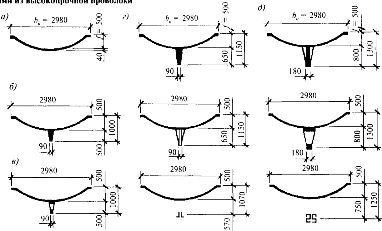
Рисунок 14.16 — Гиперболическая панель-оболочка, армированная пакетами из высокопрочной проволоки
