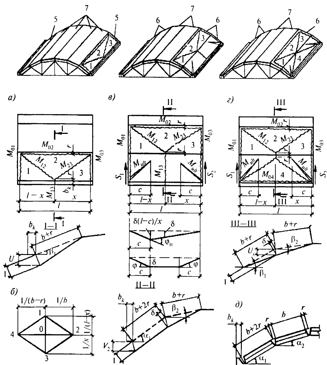
а — схемы разрушения первой грани складки и бортового элемента; б — диаграмма скоростей виртуальных перемещений; в — схема разрушений двух граний складки с изломом бортового элемента; г — то же, без излома бортового элемента; д — поперечное сечение складки у края; 1—4 — звенья в схемах разрушения; 5 — первые грани складки; 6 — первая и вторая крайние грани складки; 7 — средняя часть складки
