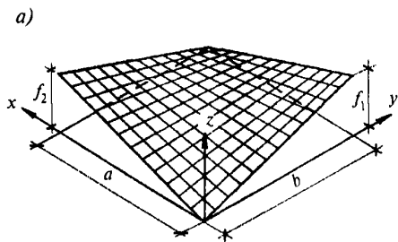
Рисунок 12.2 — Однолепестковые гипары
