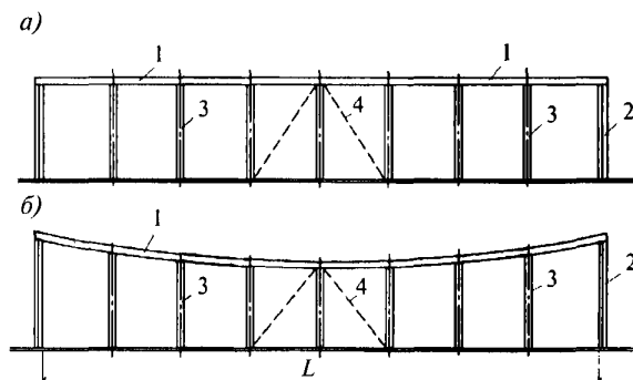
1 — опорный контур; 2 — угловые (двойные) колонны; 3 — промежуточные колонны; 4 — вертикальные связи; а — с горизонтальным контуром; б — с полигональным контуром
