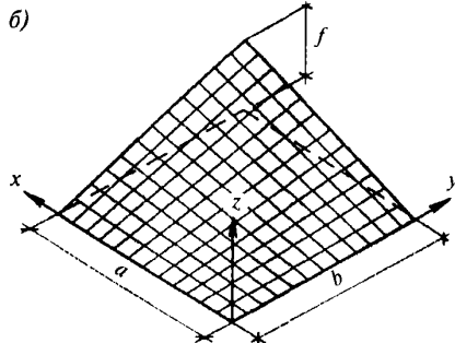
Рисунок 12.2 — Однолепестковые гипары
