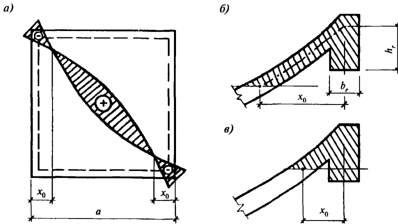
а — схема излома; б, в — схемы расположения нейтральной оси Рисунок 12.5 — К расчету оболочек, опертых по нижним углам
