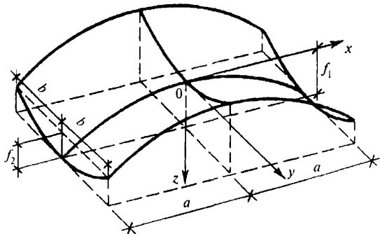
Рисунок 12.1 — Гиперболический параболоид
