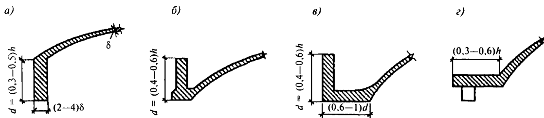
Рисунок 9.11 — Бортовые элементы
