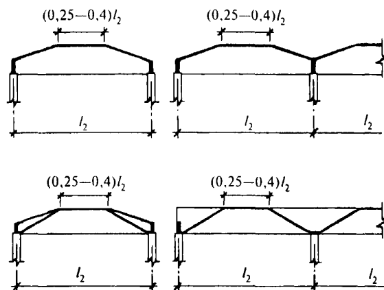
Рисунок 9.2 — Типы складчатых оболочек
