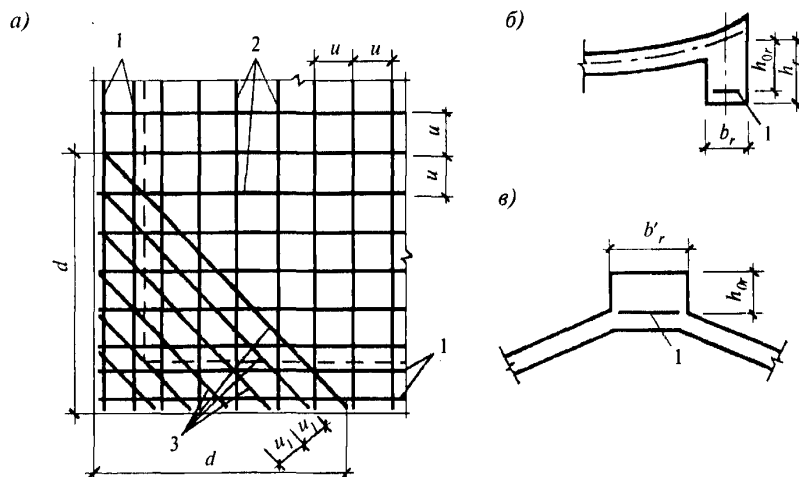
Рисунок 12.4 — Узлы гипаров
