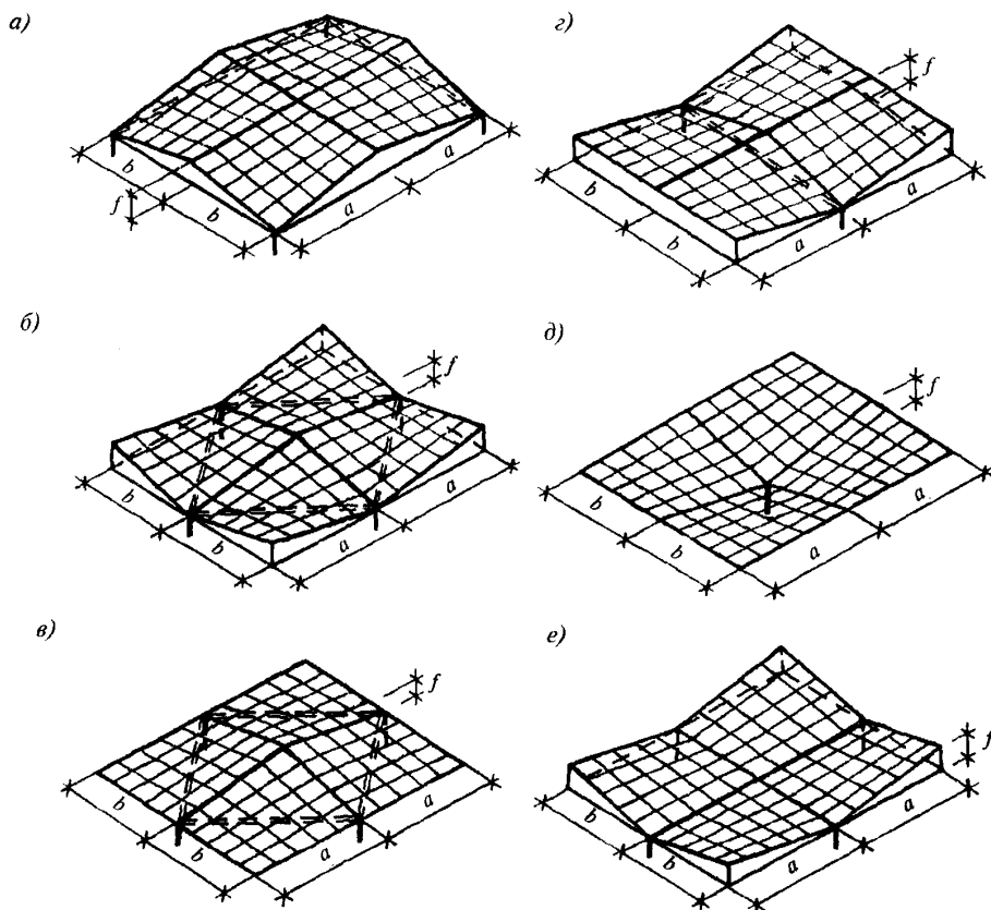
Рисунок 12.3 — Четырехлепестковые гипары
