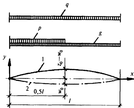
Рисунок 14.6 — Расчетная схема панели-оболочки КЖС
