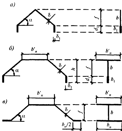
Рисунок 8.2 — Схемы поперечных сечений складок и их приведение для расчета
