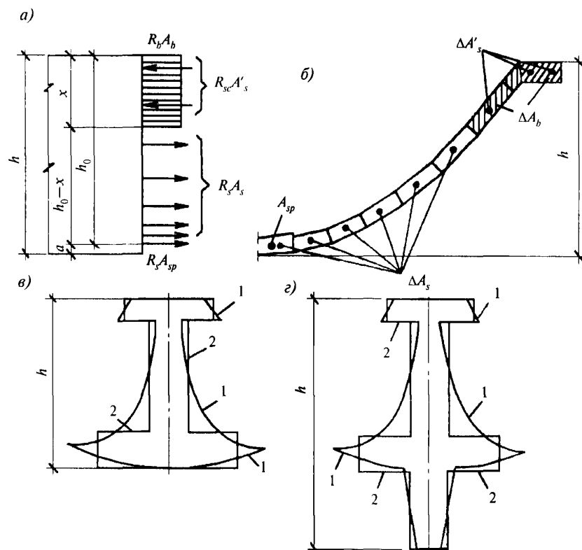
а — схема усилий в поперечном сечении изгибаемой волны; б — разбивка на элементарные площадки половины поперечного сечения; в — приведенное поперечное сечение при расчете на изгиб панели-оболочки; г — то же, килевой панели-оболочки; 1 — контур фактического приведенного сечения; 2 — то же, расчетного приведенного сечения
