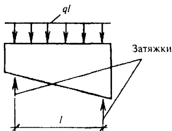
Рисунок 7.7 — Расчетная схема опорной панели
