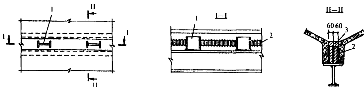
Рисунок 6.6 — Схема стыков соединений железобетонных и металлических элементов
