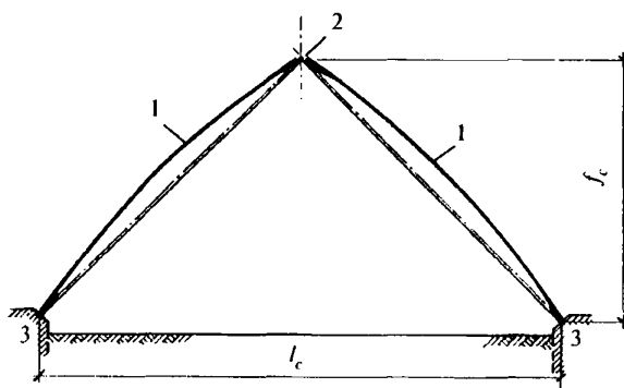
1 — панель-оболочка КЖС; 2 — ключевой шарнир; 3 — фундамент
