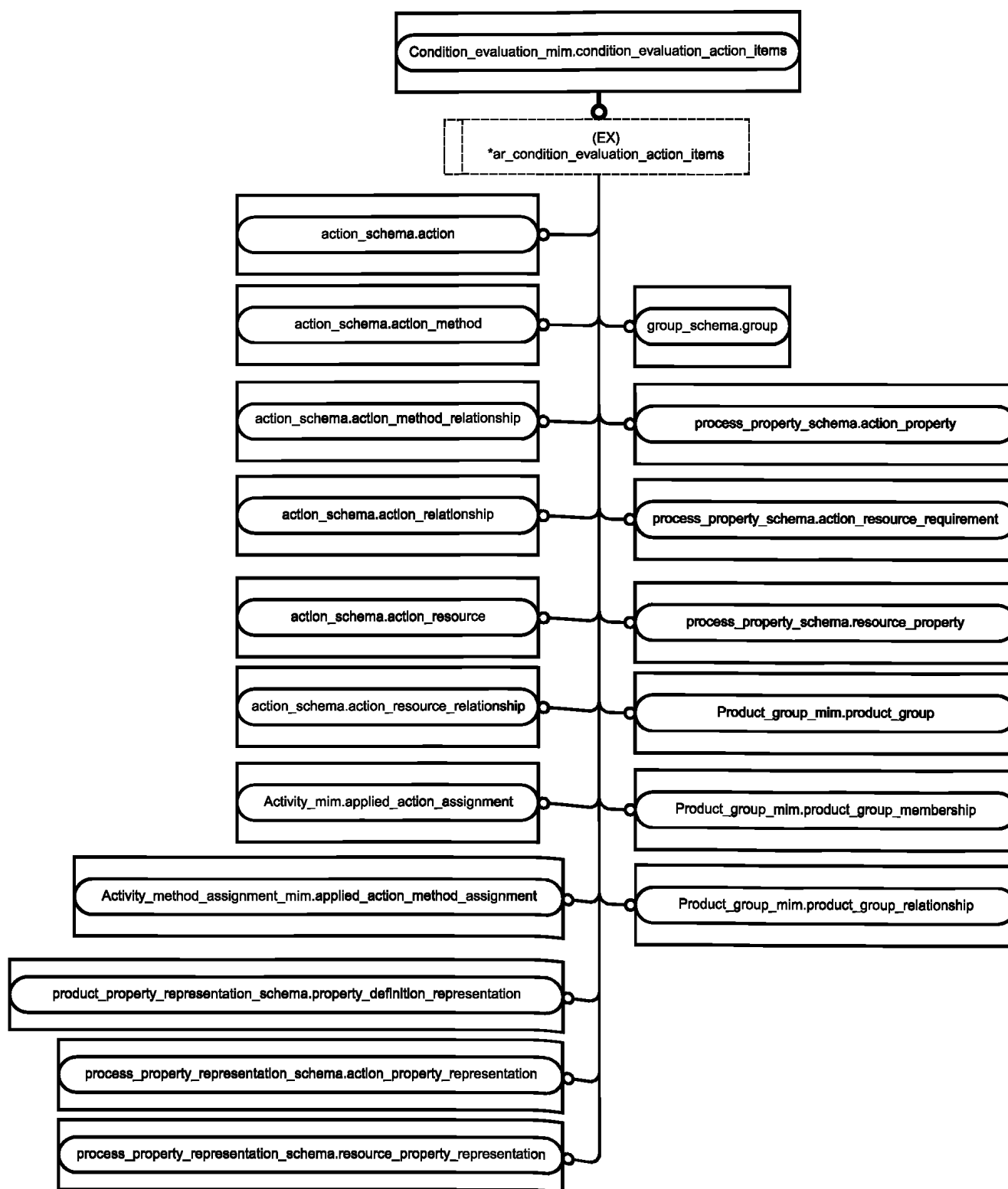
Рисунок D.3 — Представление ИММ на уровне объектов в формате EXPRESS-G (диаграмма 2 из 4)
