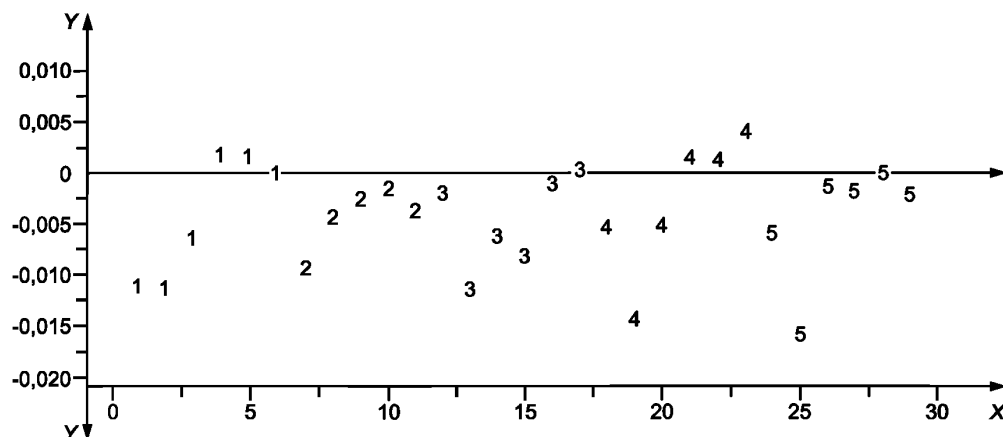
X — время, дни; Y — разность удельного сопротивления в двух конфигурациях, Ом · см; 1, ..., 5 — идентификационные номера пластин (см. таблицу 6)
