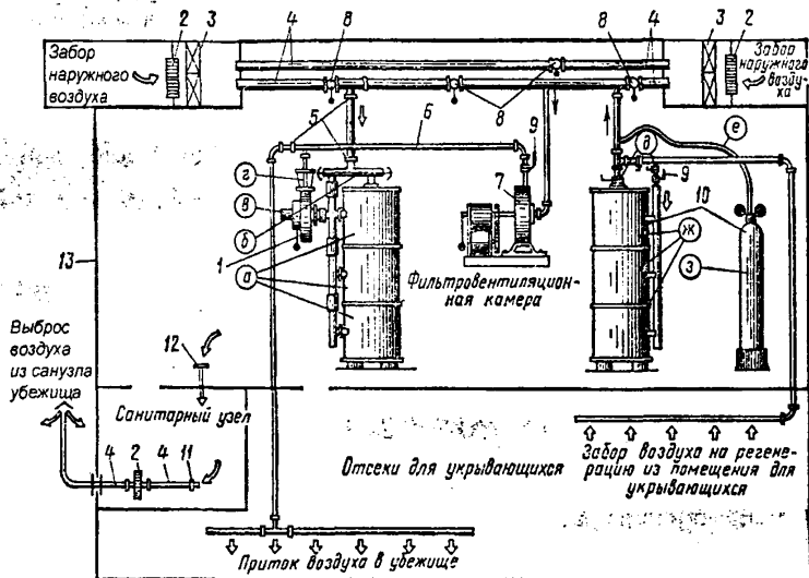
Рис. 1.23. Принципиальная схема воздухообмена убежища с фильтровентиляционным оборудованием старого образца
