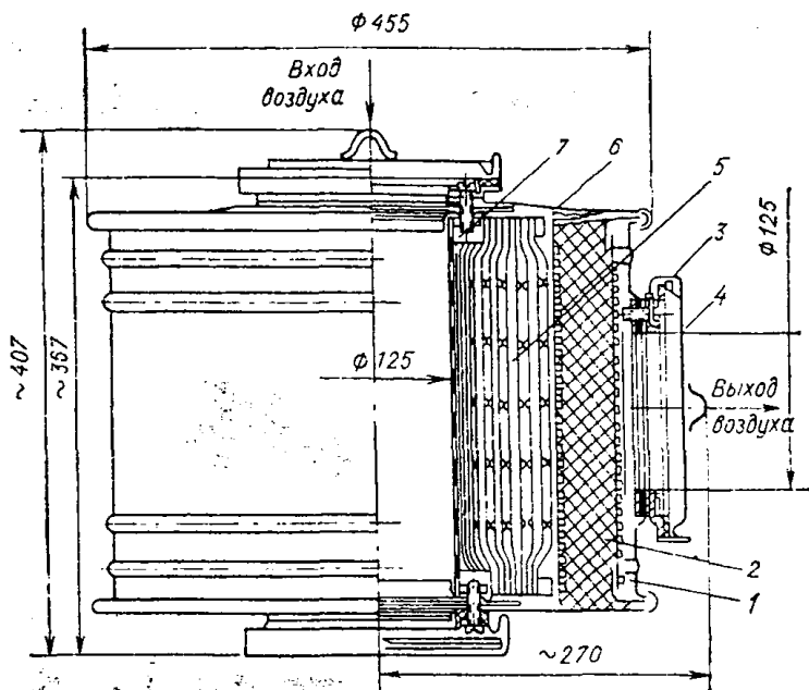
Рис. 1.19. Фильтр- поглотитель ФПУ-200
