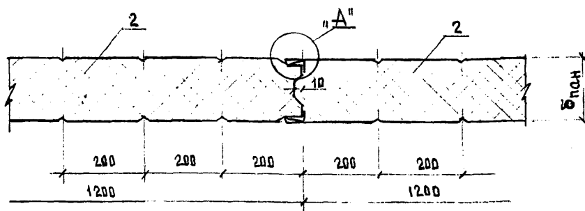
ГСИ.Рис.2. ПРОДОЛЬНЫЙ СТЫК СТЕНОВЫХ ПАНЕЛЕЙ
