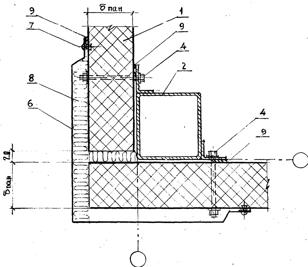
ГОС.РИС.2. СОПРЯЖЕНИЕ ПАНЕЛЕЙ В УГЛУ ЗДАНИЯ ПРИ \delta_{пан} > 150
