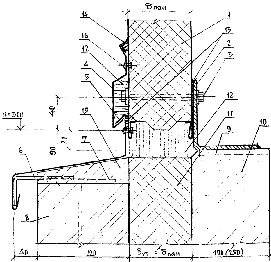
ГОСТ.РИС.1. СОПРЯЖЕНИЕ ЦОКОЛЯ СО СТЕНОВЫМИ ПАНЕЛЯМИ
