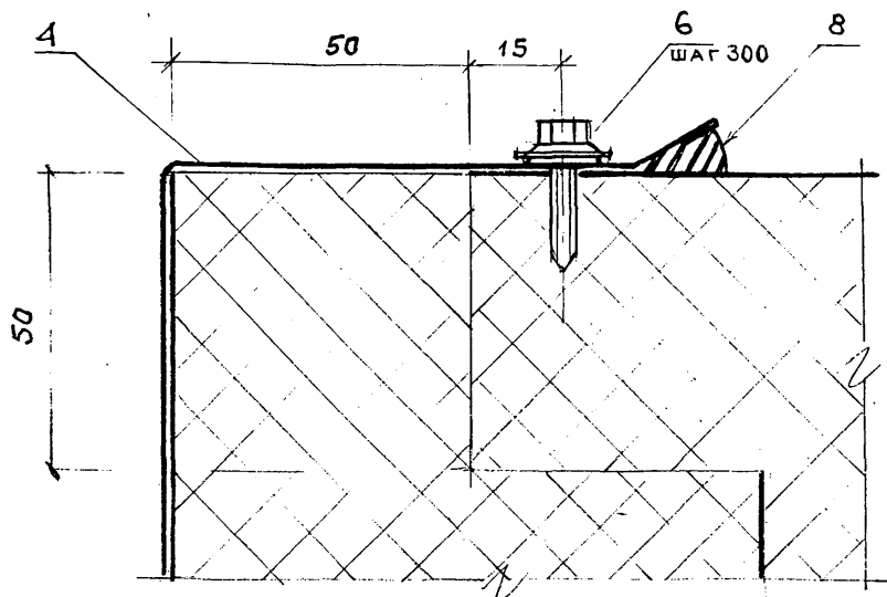
Деталь А
