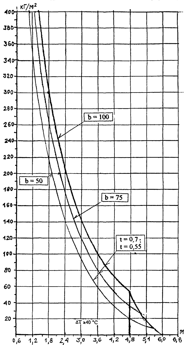
Рис 5г. Зависимость "пролет-нагрузка" для двухпролетной панели толщиной 250 мм с толщиной обшивок 0.55 ... 0.7мм b -ширина опирания в мм ; t -толщина обшивки в мм
