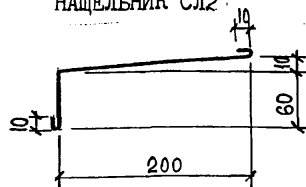
НАЩЕЛЬНИК СЛ2
