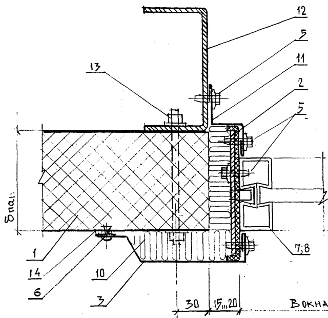
ОК 5.Рис. 2. БОКОВОЕ СОПРЯЖЕНИЕ ОКНА СО СТАЛЬНЫМИ ПЕРЕТЫТАМИ ПРИ ГОРИЗОНТАЛЬНОМ РАЗРЕЗЕ СТЕНОВЫХ ПАНЕЛЕЙ ИЛИ ПРИ МНОГОЯРУСНЫХ ОКНАХ
