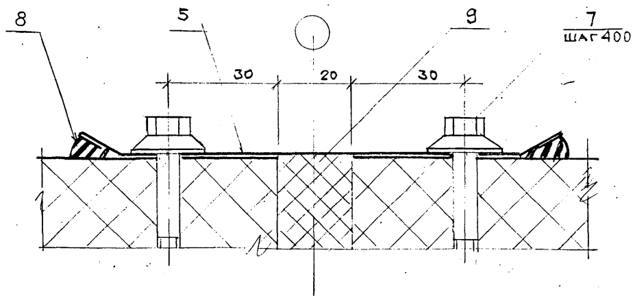
Деталь Б
