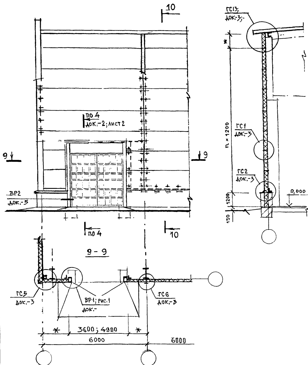
СХЕМА 16. ПРОДОЛЬНАЯ СТЕНА ИЗ ОДНОПРОЛЕТНЫХ ПАНЕЛЕЙ С ВОРОТАМИ (ВАРИАНТ С КАРНИЗОМ)
