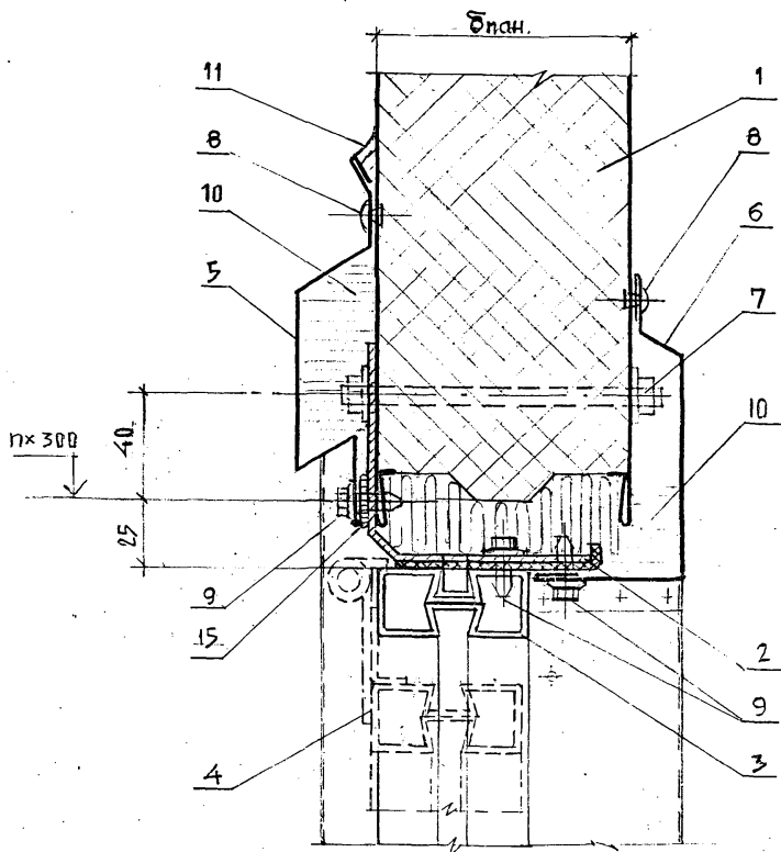
ОК 2. РИС.1. ВЕРХ ОКНА СО СТАЛЬНЫМИ ПЕРЕПЛЕТАМИ. ГОРИЗОНТАЛЬНОЕ РАСПОЛОЖЕНИЕ СТЕНОВОЙ ПАНЕЛИ
