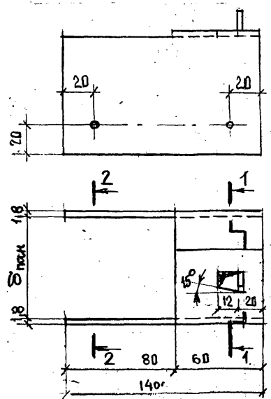
ОПОРА ОП3Д (ОПОРА ОП3П)
