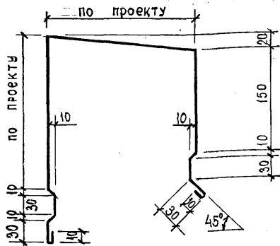
СЛИВ СЛ5
