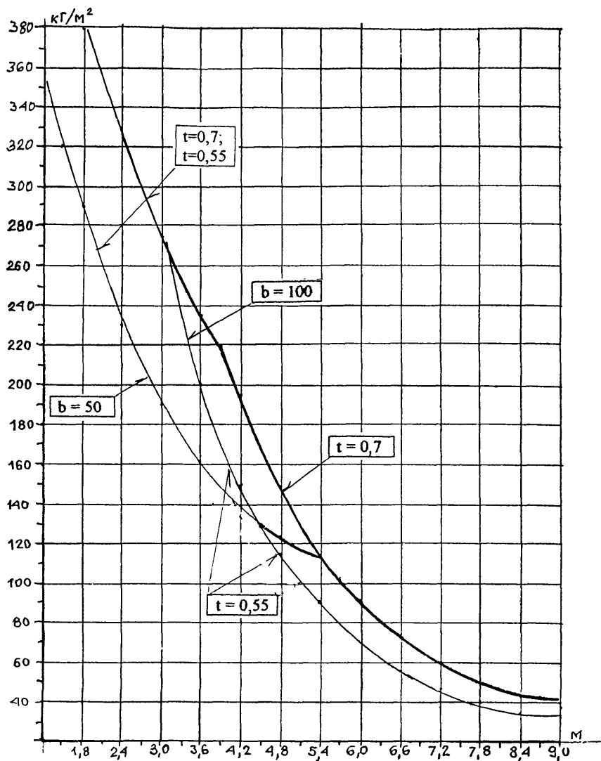
Рис 4с. Зависимость "пролет-нагрузка" для однопролетной стеновой панели толщиной 200мм b-ширина опирания в мм; t-толщина обшивки в мм
