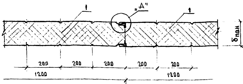
ГСИ.Рис.2. ПРОДОЛЬНЫЙ СТЫК СТЕНОВЫХ ПАНЕЛЕЙ
