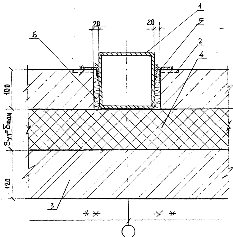
ГС 8.* РИС. 1. СОПРЯЖЕНИЕ КОЛОНН С ЦОКОЛЕМ ИЗ ЖЕЛЕЗОБЕТОННЫХ ПАНЕЛЕЙ
