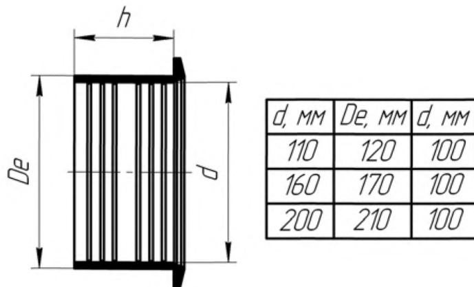
Рис. 43. Уплотнительная манжета.
