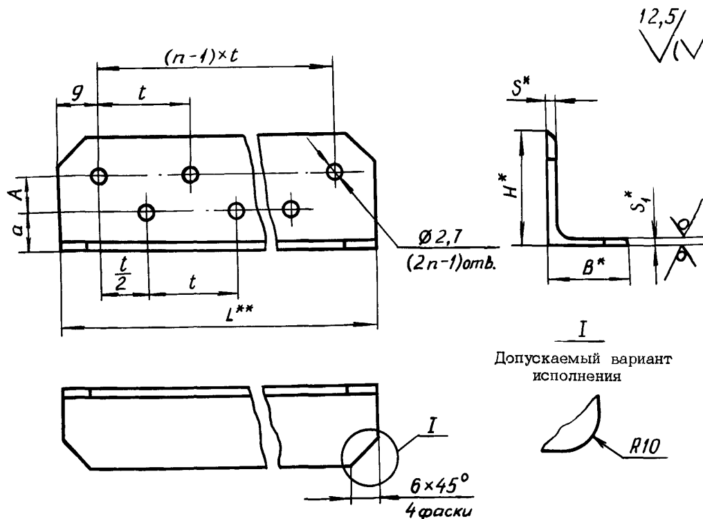
Размеры, мм
