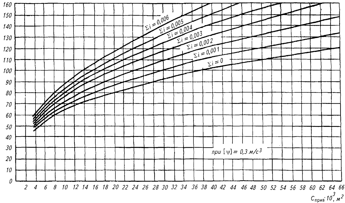
Рис. 6. Зависимости допускаемой скорости движения от приведенных параметров сопряжения C_{\text{прив}} и \Sigma i при длине прямой вставки от 15 до 25 м (включительно)
