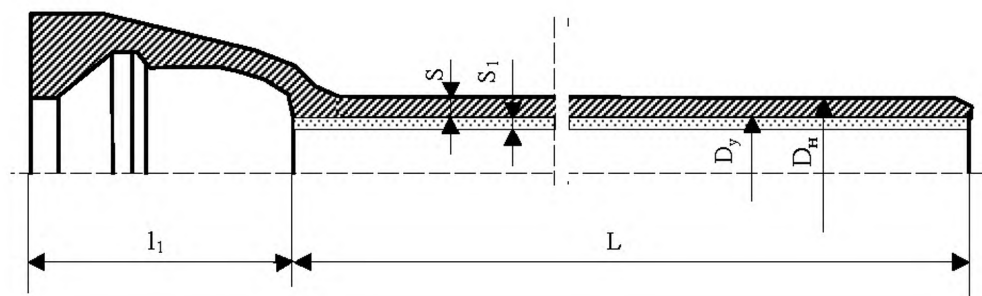
Рисунок А.1 – Труба раструбная под соединение «Универсал»
