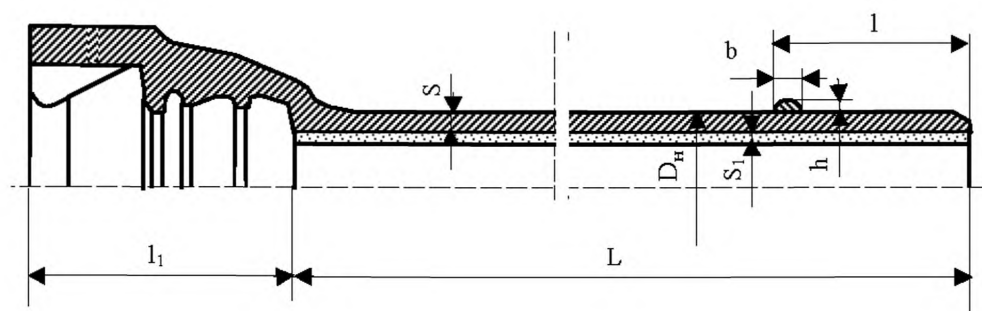
Рисунок А.3 – Труба раструбная под соединение «ВРС»
