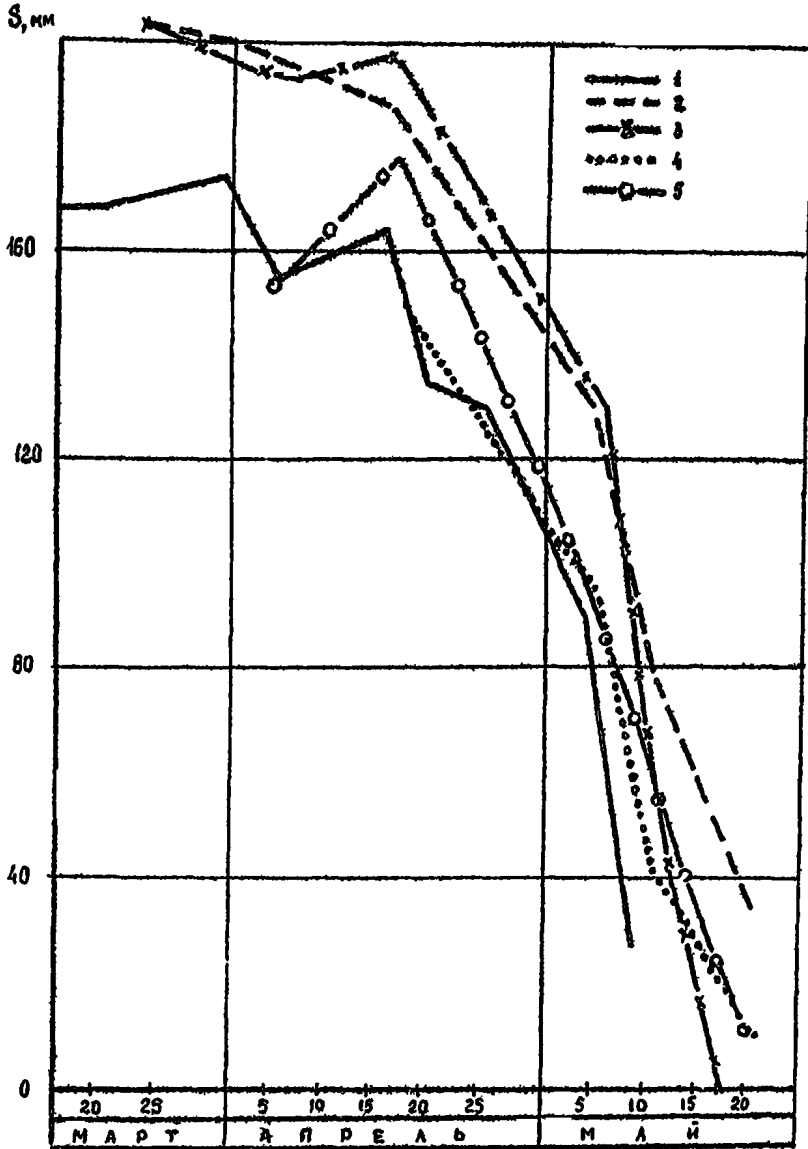
Рис. 3.2 Изменение запасов воды на поверхности водосбора Вычегды в период снеготаяния 1984 г. 1- наземные измерения, 2- авиационные измерения, 3- расчет по коэфф.стаивания, 4- расчет по \rho_{\gamma_{\text{та}}} , 5- расчет по контрольным маршрутам
