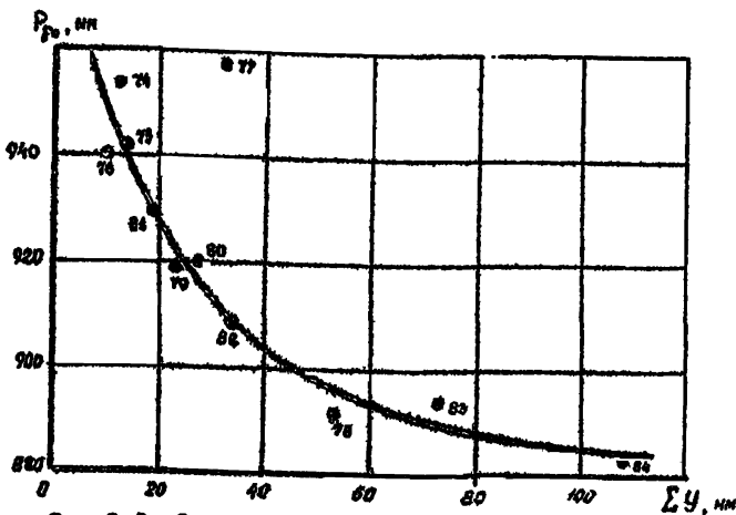
Рис. 2.3 Связь начальных уровней гамма-поля с суммарным речным стоком за октябрь и ноябрь для водосбора р. Уг
