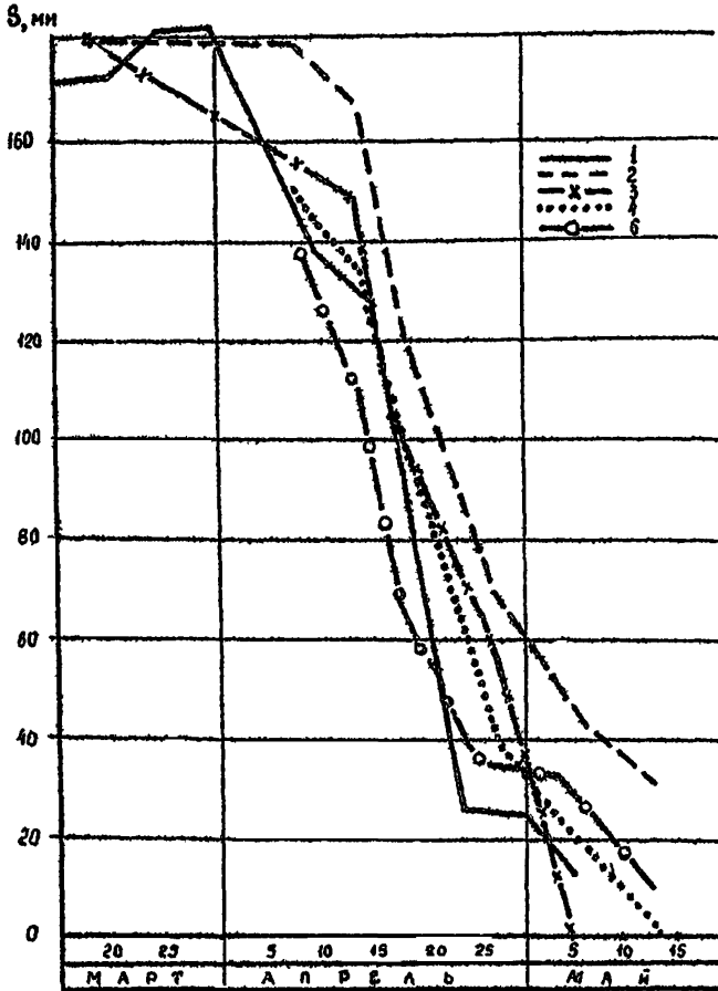
Рис.3.1 Изменение запасов воды на поверхности водосбора Сухоны в период снеготаяния 1984 г. 1- наземные измерения, 2- авиационные измерения, 3- расчет по коэф.таивания, 4- расчет по P_{субд.} , 5- расчет по контрольным маршрутам
