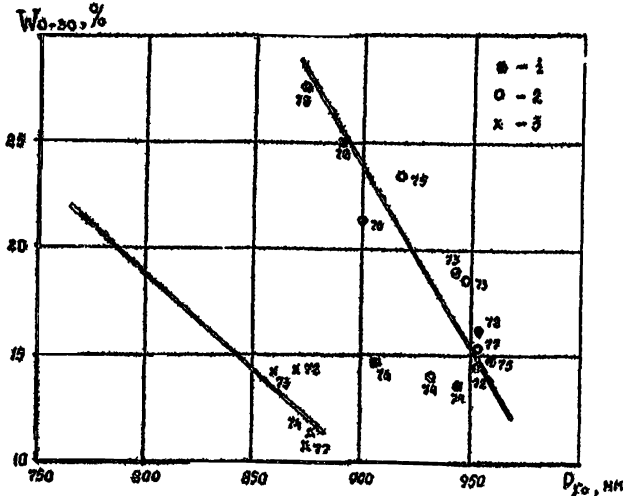
Рис. 2.1 Зависимость весовой влажности 30-см слоя почвы от начальных уровней гамма-поля 1 - водосбор Сухони, 2 - водосбор Пга, 3 - водосбор Вычегды
