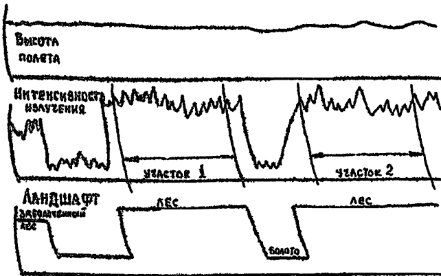
Рис. 1.1 Пример выделения участков авиационного маршрута (кольцо 7, маршрут 9, 22.10.81г.)
