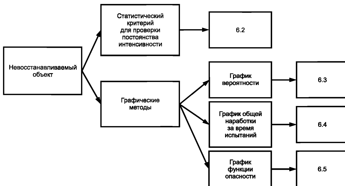
Рисунок 1 — Структура раздела 6
