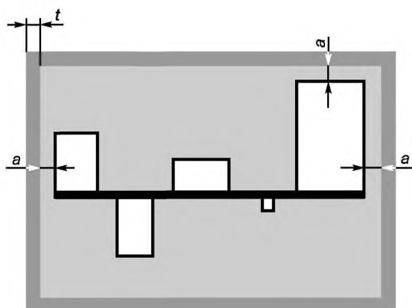
Пластмассовый корпус со всех сторон
