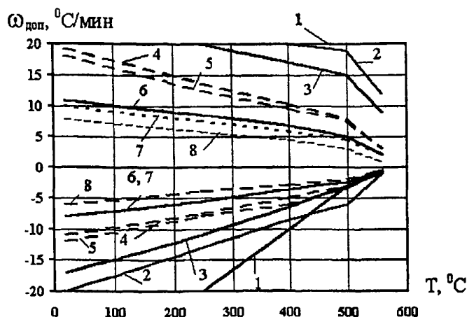
Рис.2. Допустимые скорости \omega_{\text{доп}} нагрева и расхолаживания коллекторов котлов (1 - 273×30 мм; 2 - 273×40 мм; 3 - 325×45 мм; 4 - 325×60 мм; 5 - 273×60 мм; 6 - 325×75 мм; 7 - 219×70 мм; 8 - 325×85 мм).
