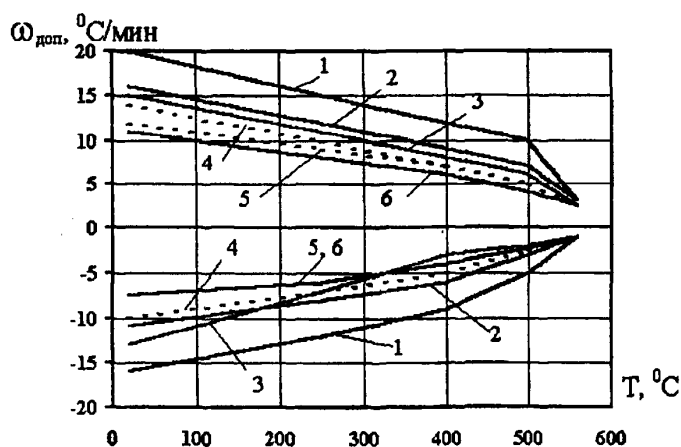
Рис.1. Допустимые скорости \omega_{\text{доп}} прогрева и расхолаживания паропроводов свежего пара (1 - 194 \times 36 мм; 2 - 245 \times 45 мм; 3 - 219 \times 32 мм; 4 - 219 \times 52 мм; 5 - 325 \times 60 мм; 6 - 275 \times 62,5 мм).
