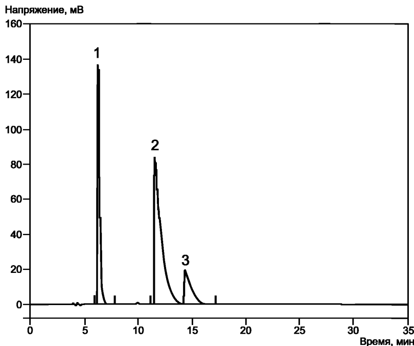
Рисунок 3 — Хроматограмма калибровочного раствора А
