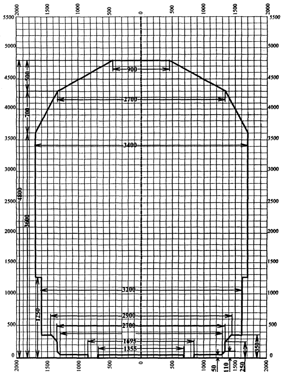
Рис. П.18.5. Габарит погрузки железных дорог КНР (КЖД) – коля 1435 мм
