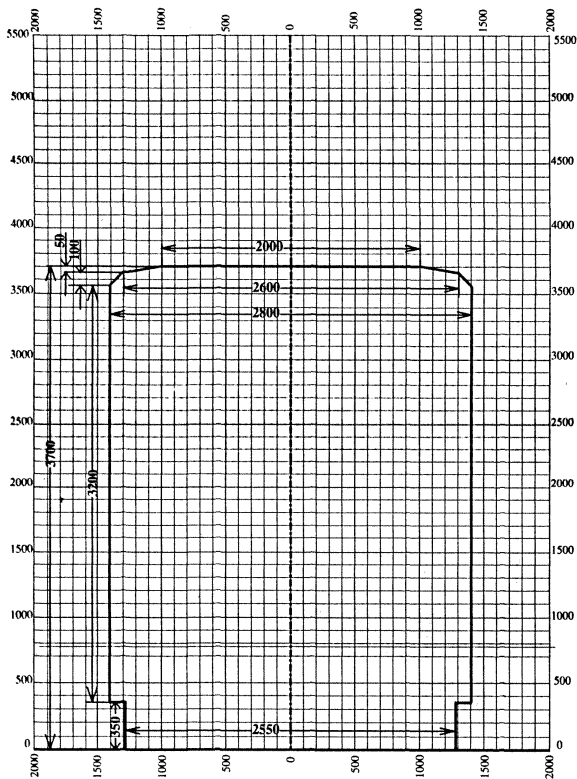
Рис. П.18.6. Габарит погрузки железных дорог СРВ (ДСВН) – кося 1000 мм
