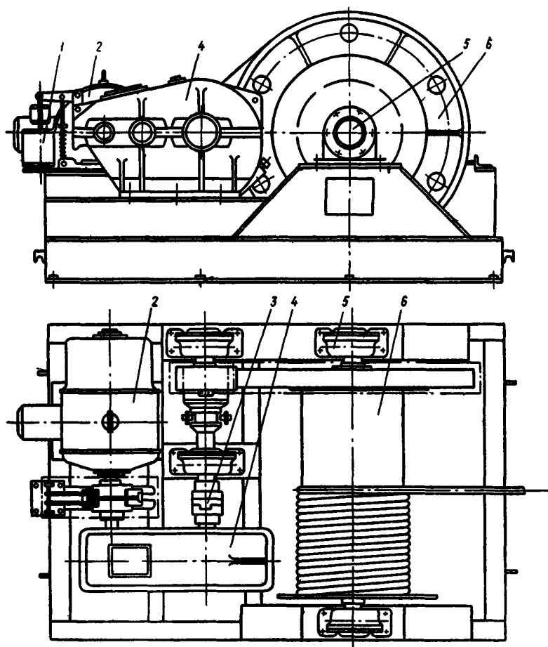
Рис. 5. Электрическая лебедка
