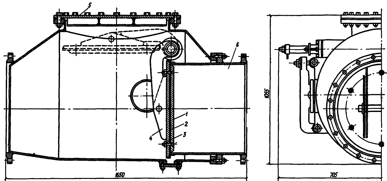
Рис 6. Обратный клапан
