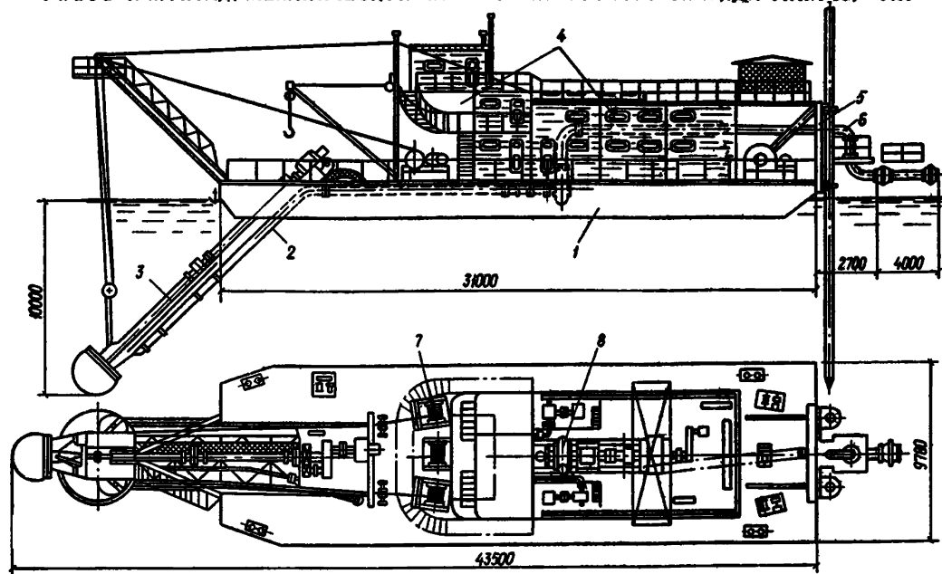
Рис. 1. Общий вид землесосного снаряда типа 350-50Л
