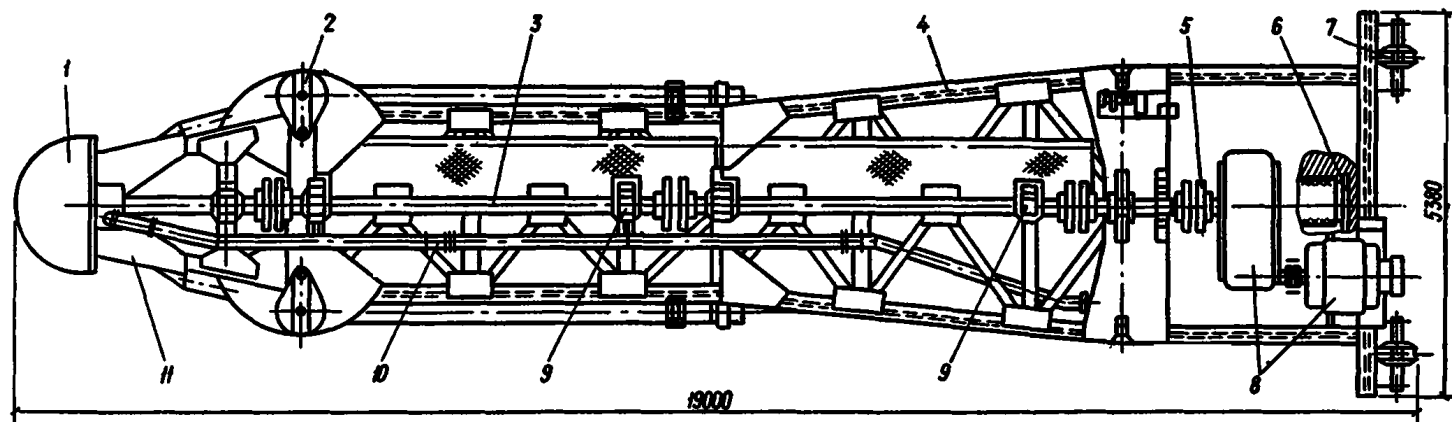
Рис. 4. Рыхлитель землесосного снаряда типа 350-50Л
