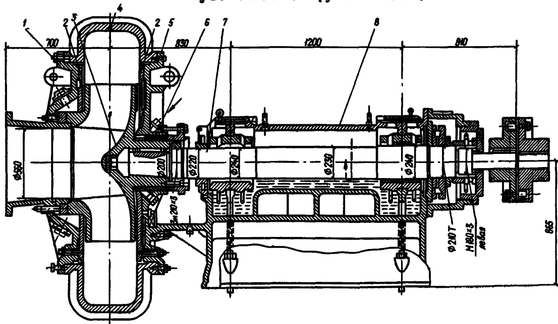
Рис. 3. Грунтовый насос типа 20P-11M .
