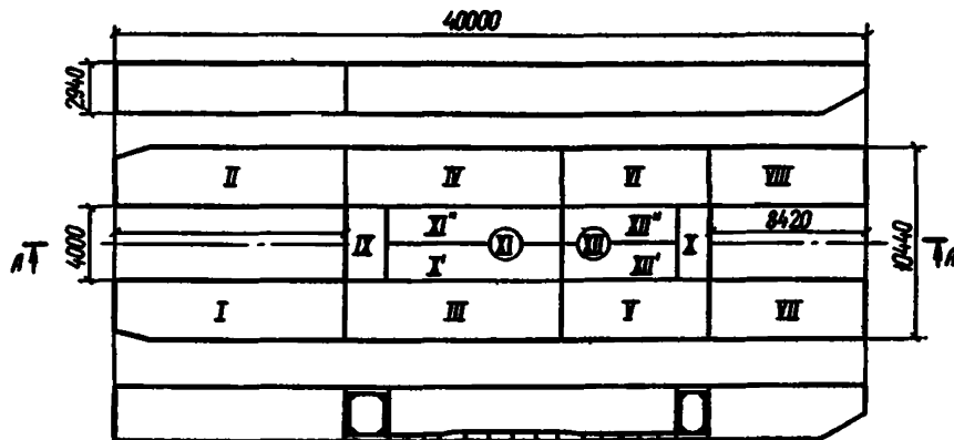
Рис. 2. Корпус землесосного снаряда типа 500-60МН
