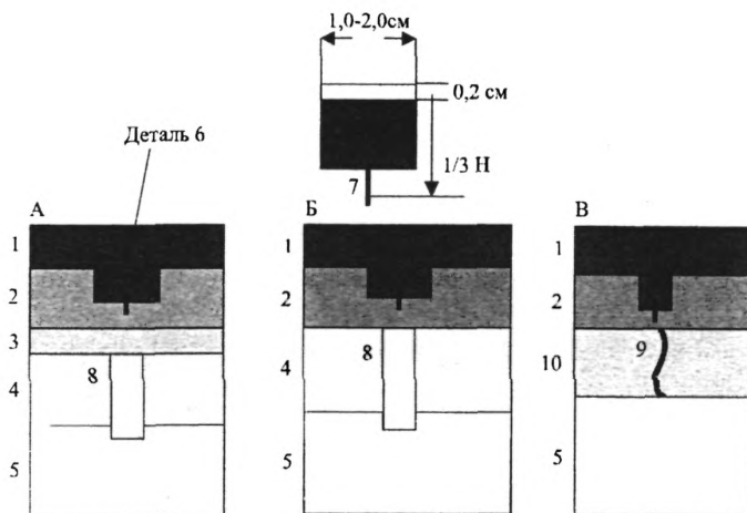
Схема нарезки «температурного шва» в нижнем слое асфальтобетонного покрытия:
