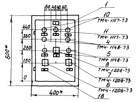
Вид на внутренние плоскости (развернуто)
