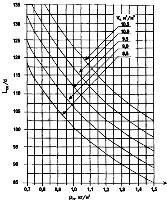
Рис.6. Номограмма для нахождения отношения стехиометрической длины факела к диаметру выходного сопла L_{ox}/d при плотности сжигаемой смеси \rho и теоретическому удельному расходу воздуха V_0
