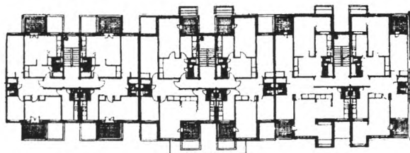
План 2-го этажа
