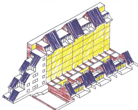
Пирамидальное построение в поперечном направлении
