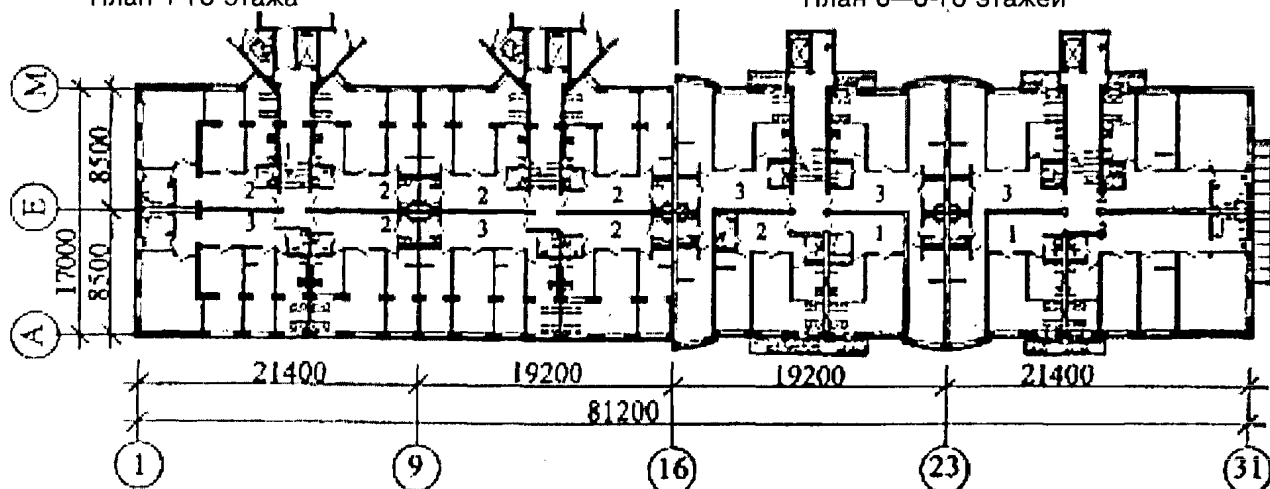
Схема каркаса. План 1—5-го этажей
