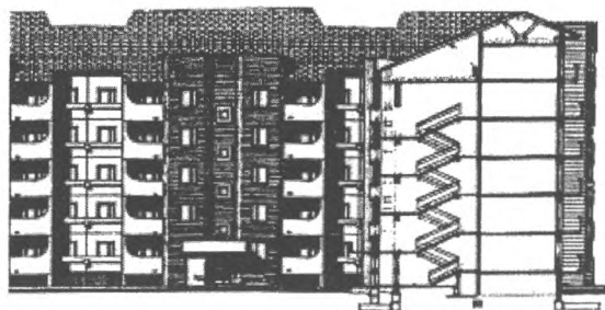
Фрагмент фасада и разрез
