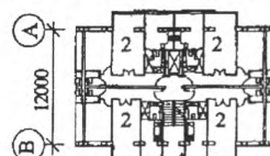
План 7-го этажа рядовой секции
