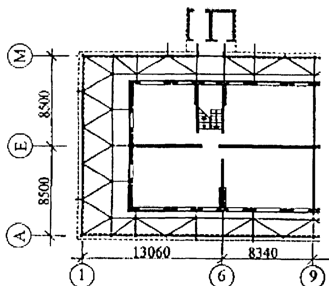
Схема каркаса. План 1—5-го этажей
