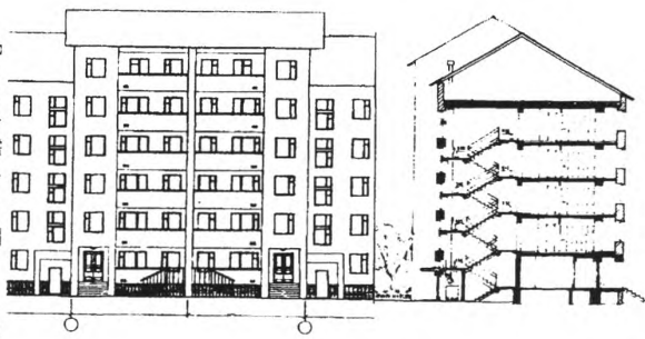
Фрагмент фасада и разрез
