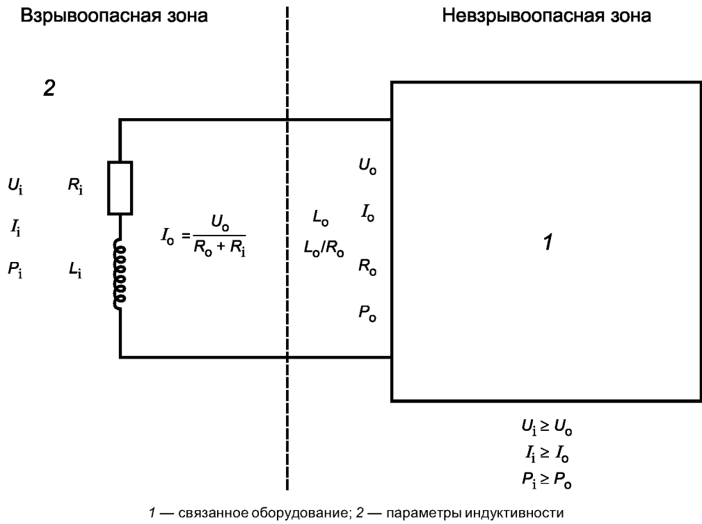
Рисунок D.1 — Типичная индуктивная цепь
