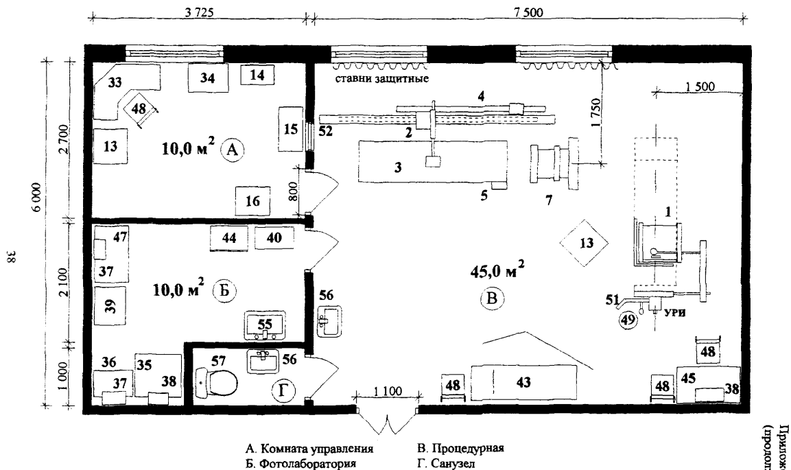
Рис.3.2. Рентгенологический кабинет для общих исследований на 3 рабочих места
