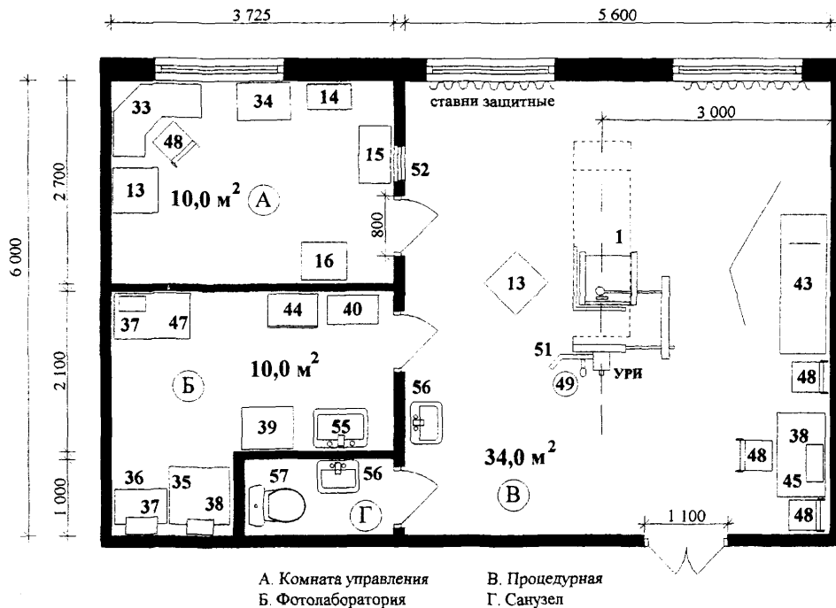
Рис.3.1. Рентгенологический кабинет с универсальным рентгеновским аппаратом
