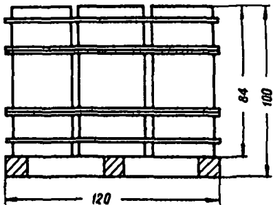
Рис. 5. Грузы катно-бочковые Общая масса подъема груза 4650 кг (6 мест)
