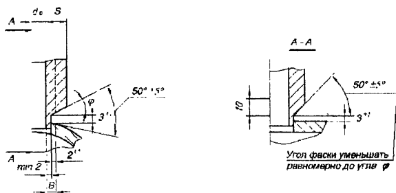
B - припуск на обработку резаньем
