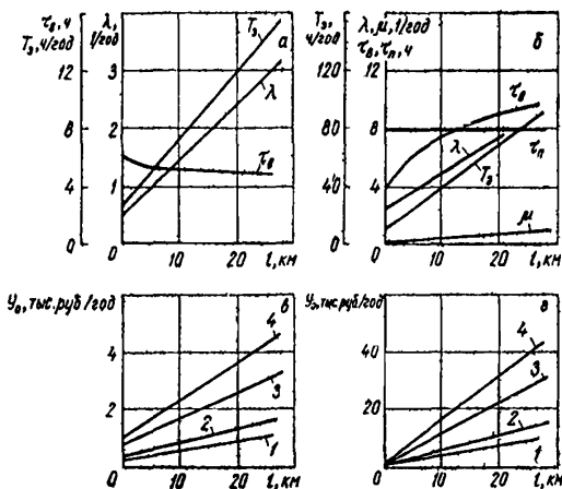
Рис. 12. Пределы изменения показателей надежности схемы 4 без РП и соответствующих ущербов:
