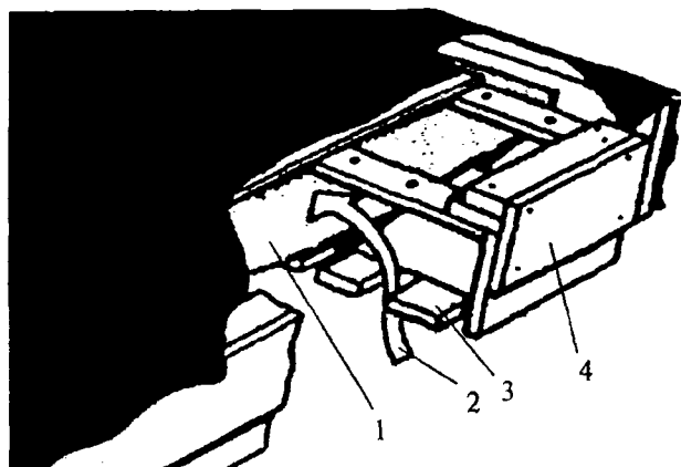
1 — антиконденсатная пленка; 2 — движение воздуха; 3 — зашивка карниза; 4 — карнизная доска
