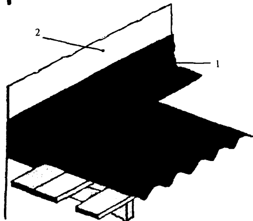
Рисунок 16 — Устройство примыкания к стене
