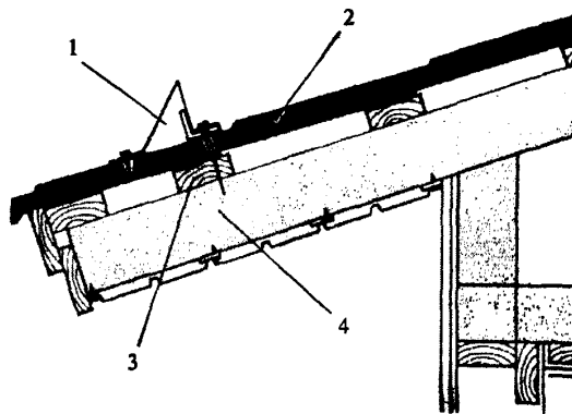
Рисунок 16 — Устройство примыкания к стене
