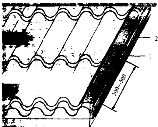
Рисунок 14 — Устройство ендовы
