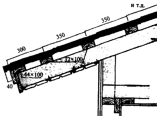
Рисунок 5 — Устройство обрешетки
