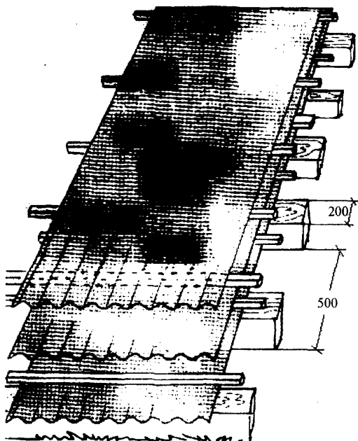
Рисунок 3 — Хранение металлочерепицы
