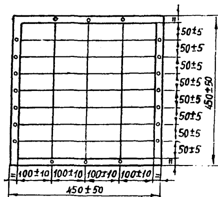
Рисунок 1. Общий вид испытательного стенда
