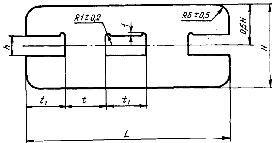
Развертка
