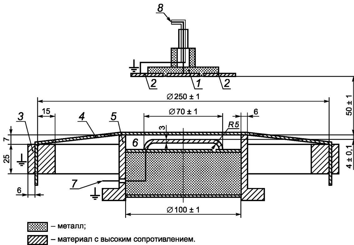
1 — датчик для измерения поля; 2 — защитное кольцо; 3 — зажимное кольцо для образца; 4 — образец для испытаний; 5 — опорное кольцо; 6 — электрод для создания поля; 7 — электропровод для соединения с генератором напряжения; 8 — электропровод для соединения с усилителем заряда
