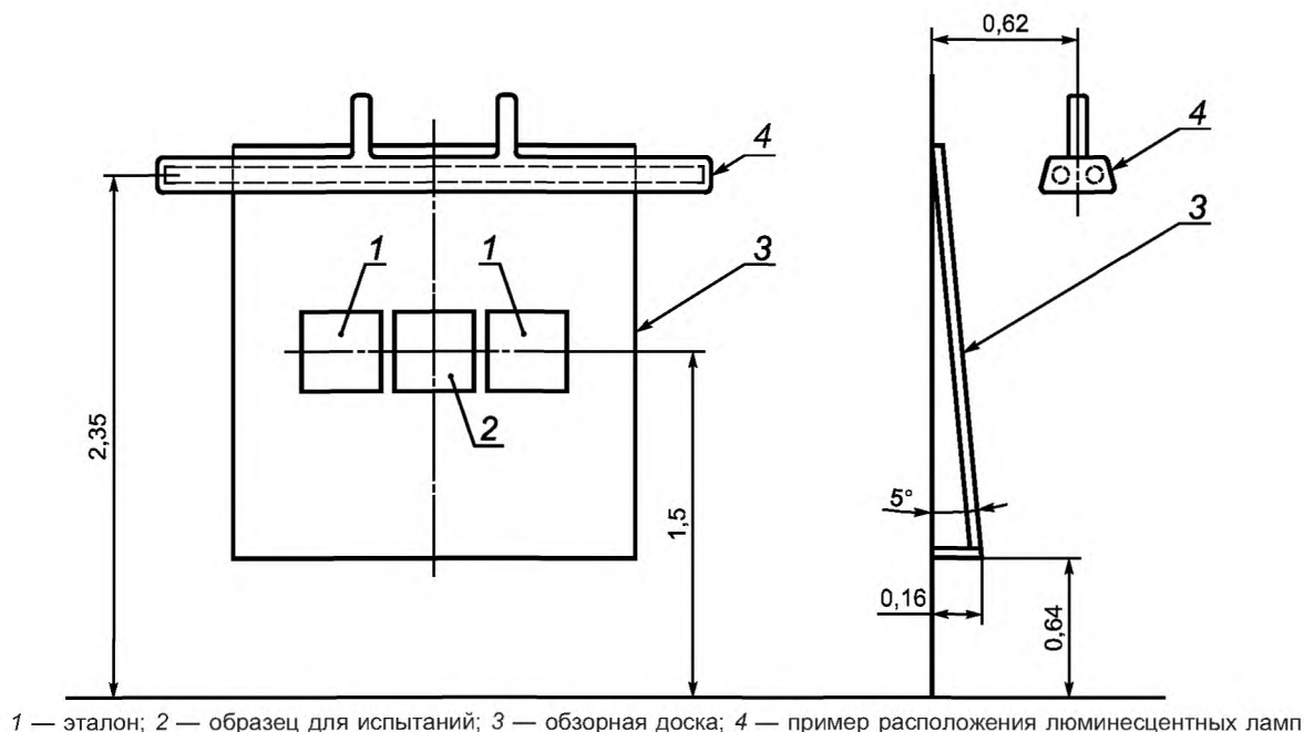
Рисунок 1 — Осветительное оборудование для просмотра образцов для испытаний
