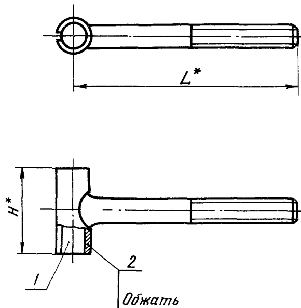
Размеры, мм
