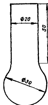
Рис. 13. Колба из туго- плавкого стекла
