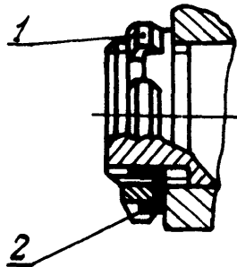
1 - гайка; 2 - шайба
