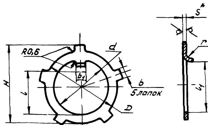
Исполнение 1
