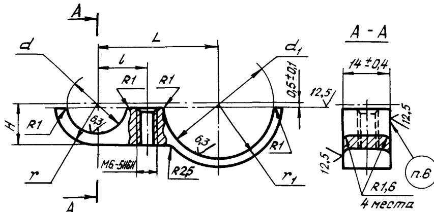
Размеры, мм
