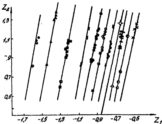
Рис. 2. Прогнозирование коэффициента гидравлического сопротивления \lambda при движении суспензий методом главных компонент: \circ - 6 %; \triangle - 10 %; \blacksquare - 15 %; \blacklozenge - 18 %; \bullet - 21 %; \circ - 23 %; \blacktriangle - 25 %; \blacktriangle - 29 %; \bullet - 31 %; \times - 34 %
