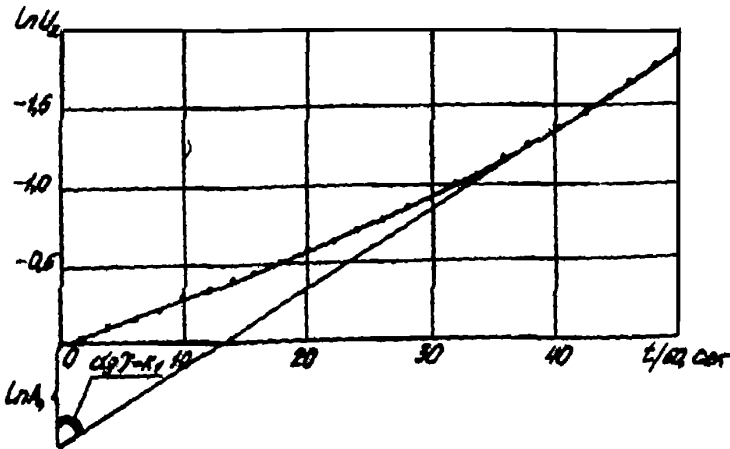
Рис. 22. Зависимость температуры от времени при \epsilon = 10\%
