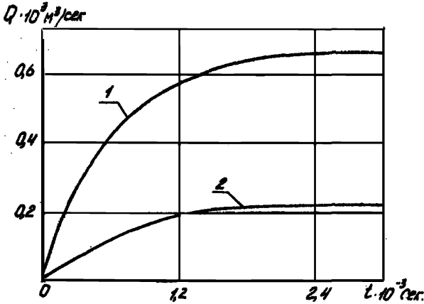
Рис. 26. Кривые восстановления расхода при постоянном перепаде давления
