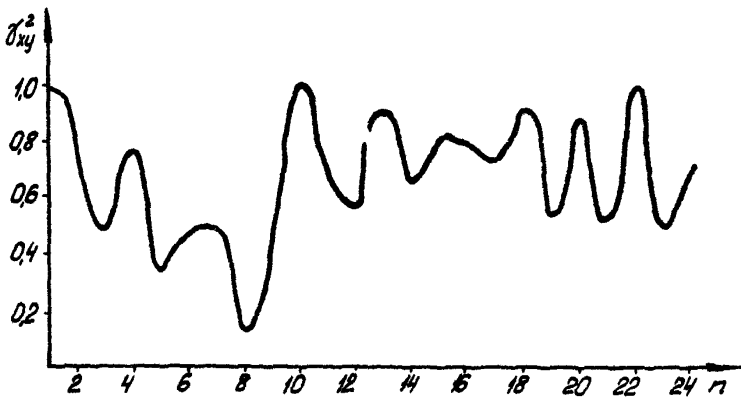
Рис.15. Распределение оценок функции когерентности производительности нефтепровода по воде и окружающей среде по частотам
