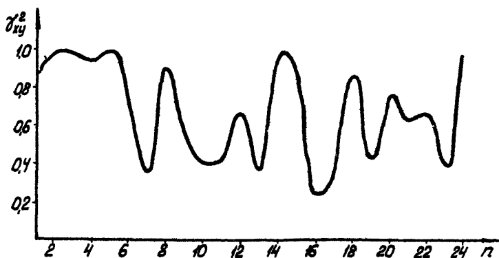
Рис.10. Распределение оценок функций когерентности производительности нефтепровода по жидкостям и нефти по частотам
