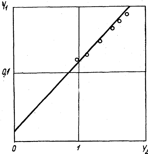
Рис. 28. Оценка гидродинамической характеристики среды методом модулирующих функций
