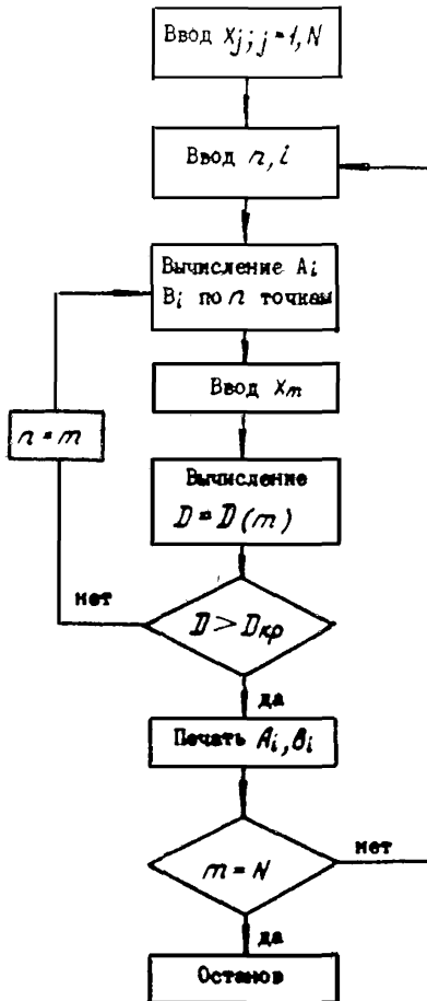
Рис.16. Блок-схема реализации возрастания дисперсии D модели с внешним воздействием
