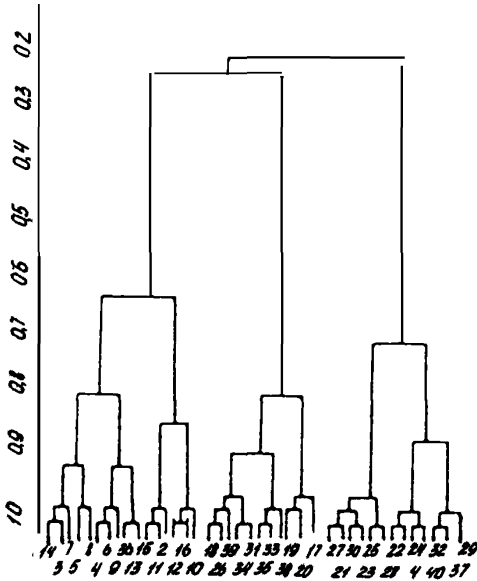
Рис. 3. Дендрограмма
