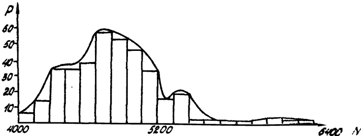
Рис. 6. Гистограмма производительности нефтепровода по воде
