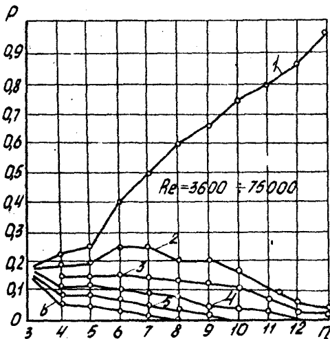
Рис. 16. Изменение вероятности P в процессе проведения эксперимента для зависимостей 1 - (2.8); 2 - (3.3); 3 - (3.1); 4 - (3.2); 5 - (3.4); 6 - (3.5)
