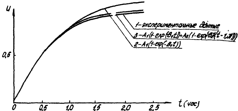
Рис. 19. Процесс восстановления температуры по эксперименту и расчетам
