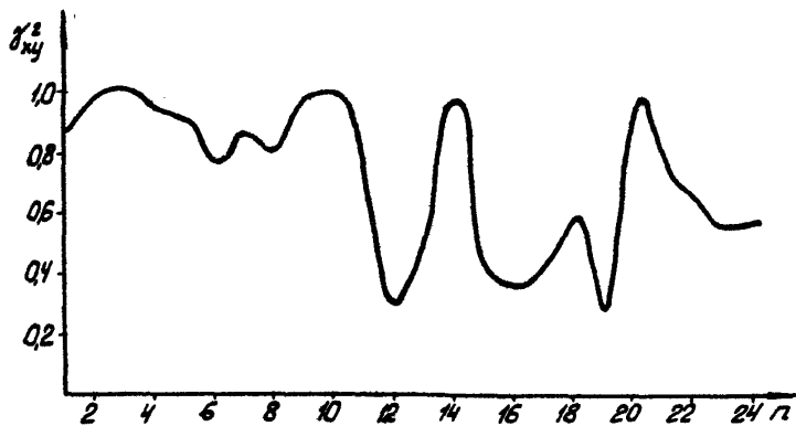
Рис.11. Распределение оценок функции когерентности производительности нефтепровода по жидкостям и воде по частотам
