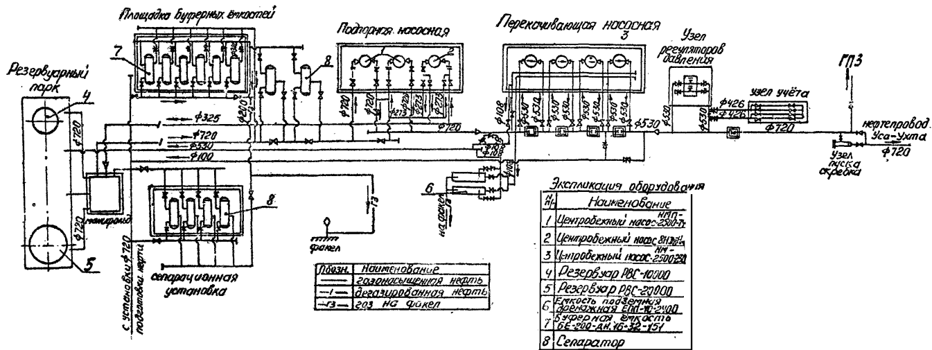
Рис.2. Принципиальная технологическая схема головной НПС "Уса"
