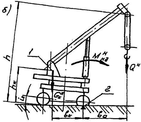
1.-центр тяжести крана ; 2.-ребро опрокидывания Черт. 1
