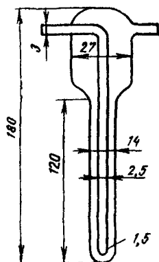
Рис. 9. Погло- тительный прибор Зайцева
