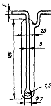
Рис. 11. Погло- тительный прибор Петри
