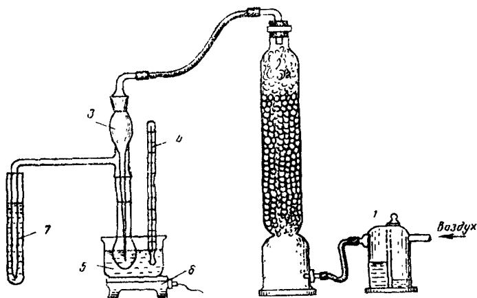
Рис 16. Приборы для разрушения хлорорганических ядохимикатов
