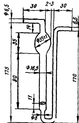
Рис. 3. Поглощительный прибор с пористой пластинкой
