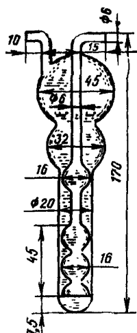
Рис. 10. Погло- тительный прибор Рихтера
