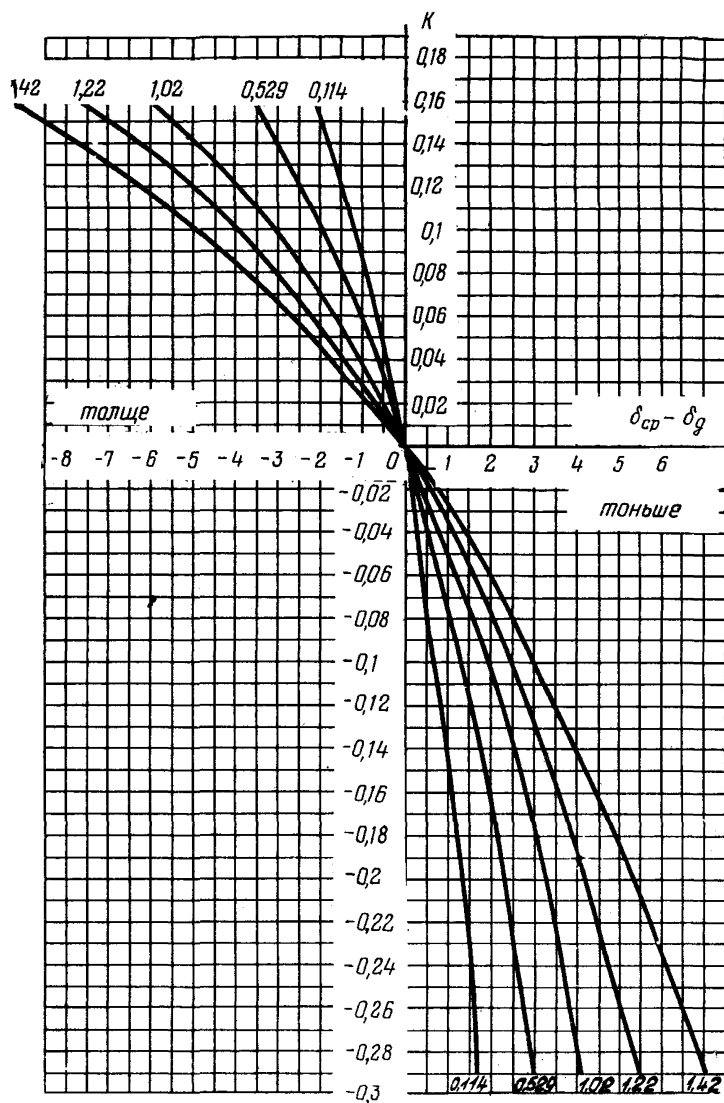
Рис.4. Зависимость K от разности между средней ( \delta_{ср} ) и действительной ( \delta_d ) толщиной стенки трубы
