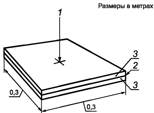
Рисунок 4 — Фантом для способа экспонирования I
