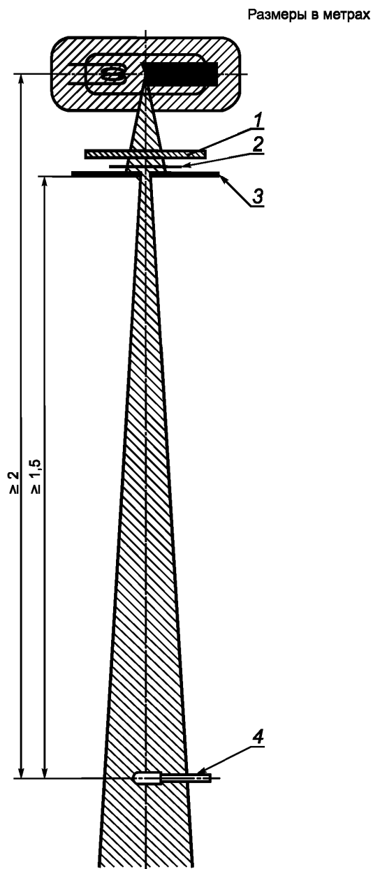
Рисунок 5 — Геометрическая схема устройства для проверки качества излучения для способов экспонирования I, II, III и IV
