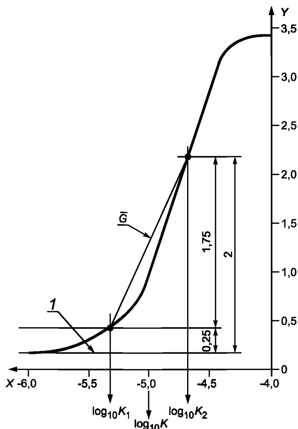
Рисунок 3 — Характеристическая кривая
