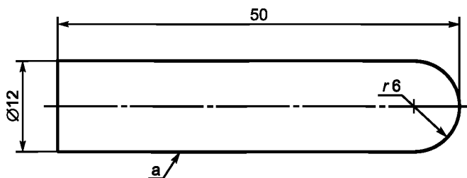
а) Испытательный палец
