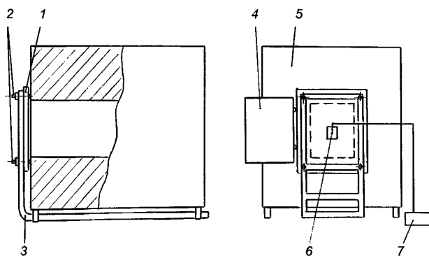
1 — прижимное устройство, 2 — крепеж образца, 3 — держатель образца, 4 — дверь камеры, 5 — электропечь, 6 — образец с термоэлектрическими преобразователями, 7 — измеритель температуры
