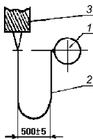
1 — контрольный груз; 2 — испытываемый образец; 3 — опора
