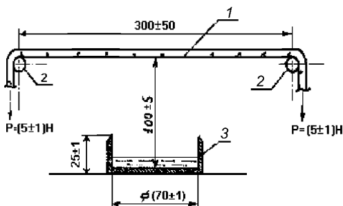
1 — образец веревки; 2 — опоры; 3 — емкость для горючего
