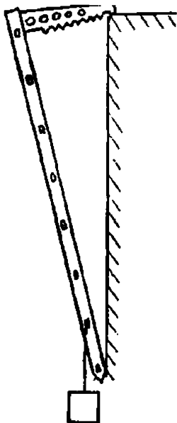
Рисунок 15 — Схема испытания крюка штурмовой лестницы на прочность
