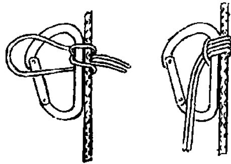
Рисунок 11 — Карабинный узел
