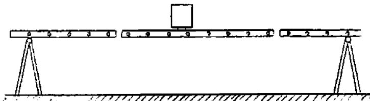
Рисунок 1 — Схема установки лестницы на опоры
