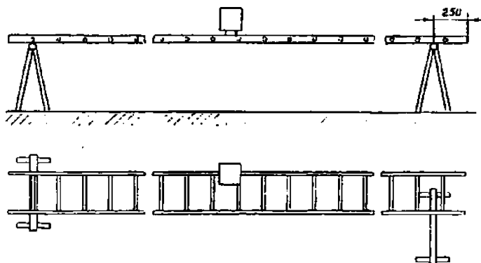
Рисунок 3 — Схема установки или подвески контрольного груза
