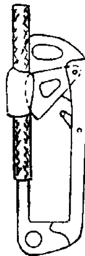
Рисунок 9 — Жумар
