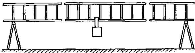
Рисунок 2 — Схема подвески контрольного груза
