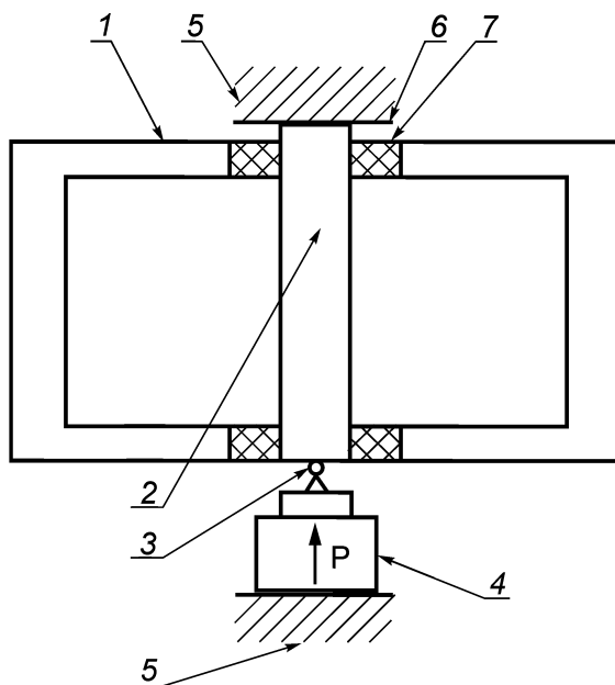
Рисунок Б.1 — Принципиальная схема установки для огневых испытаний стальной колонны под нагрузкой».
